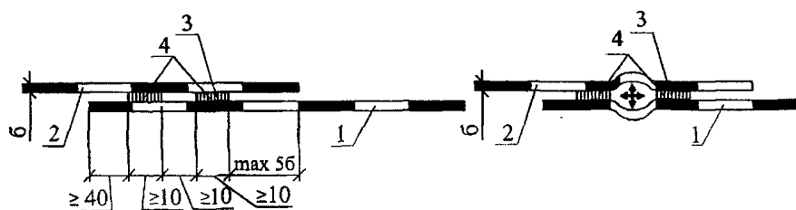
Рис 5. Испытание сварного шва с испытательным каналом
