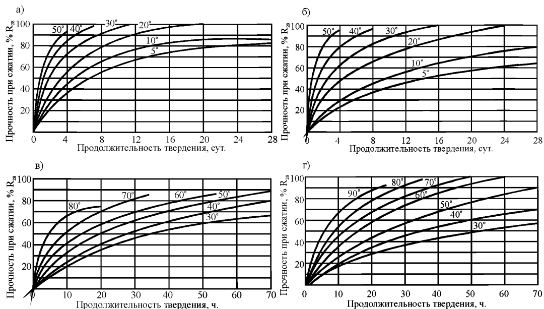
Рисунок 8 – Кривые набора прочности бетоном при различных температурах его выдерживания
