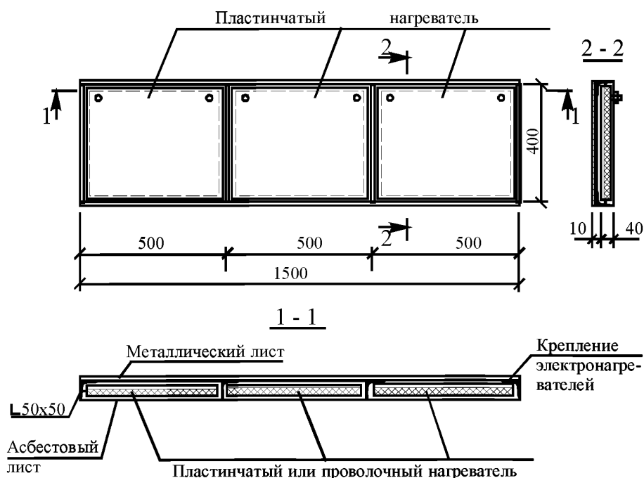
Рисунок 14 – Расстановка нагревателей на стальных щитах опалубки
