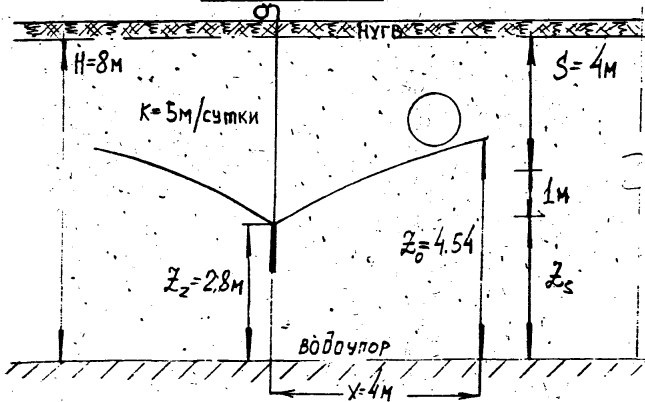
Расчетная схема
