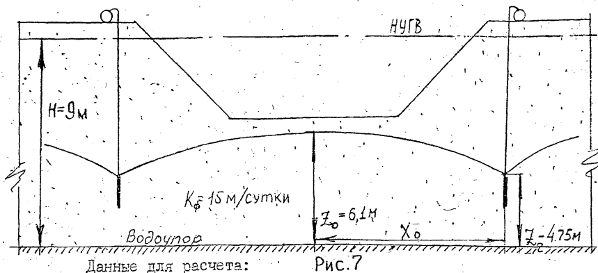
Расчетная схема
