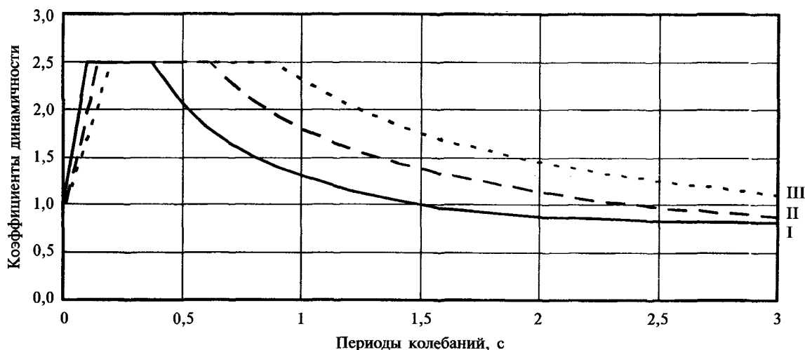
Рис. 2. Значение коэффициента динамичности \beta
