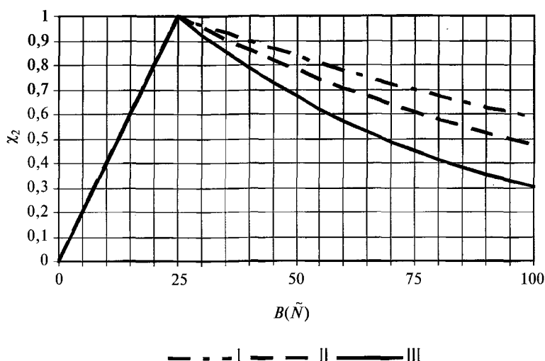
Рис. В.3. Графики нормированных функций \chi_2(B) , B , м — наименьший размер сооружения в плане
