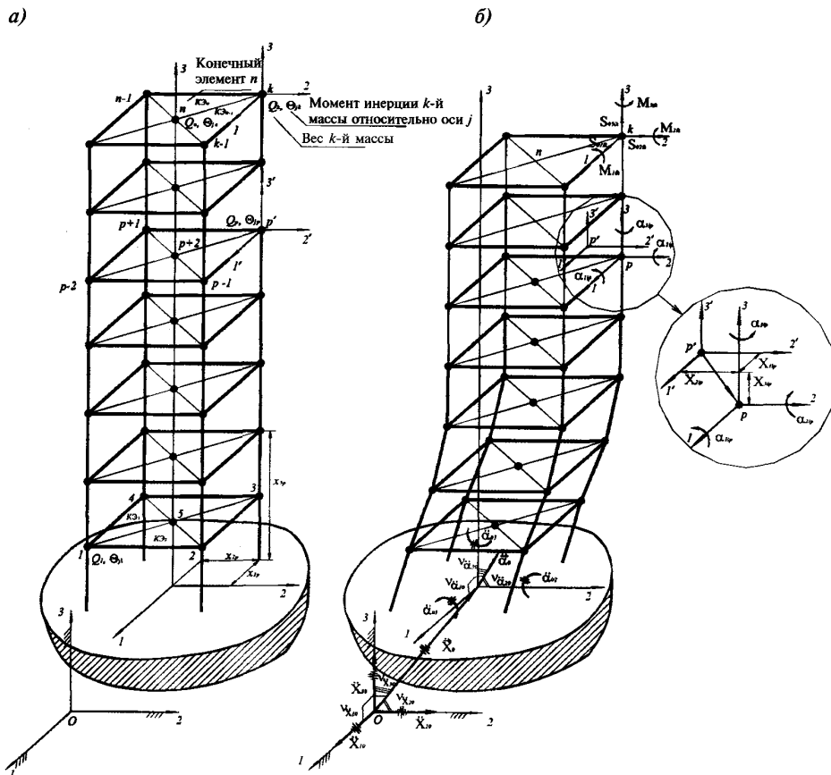
Рис. В.1. Пространственная расчетная динамическая модель сооружения
