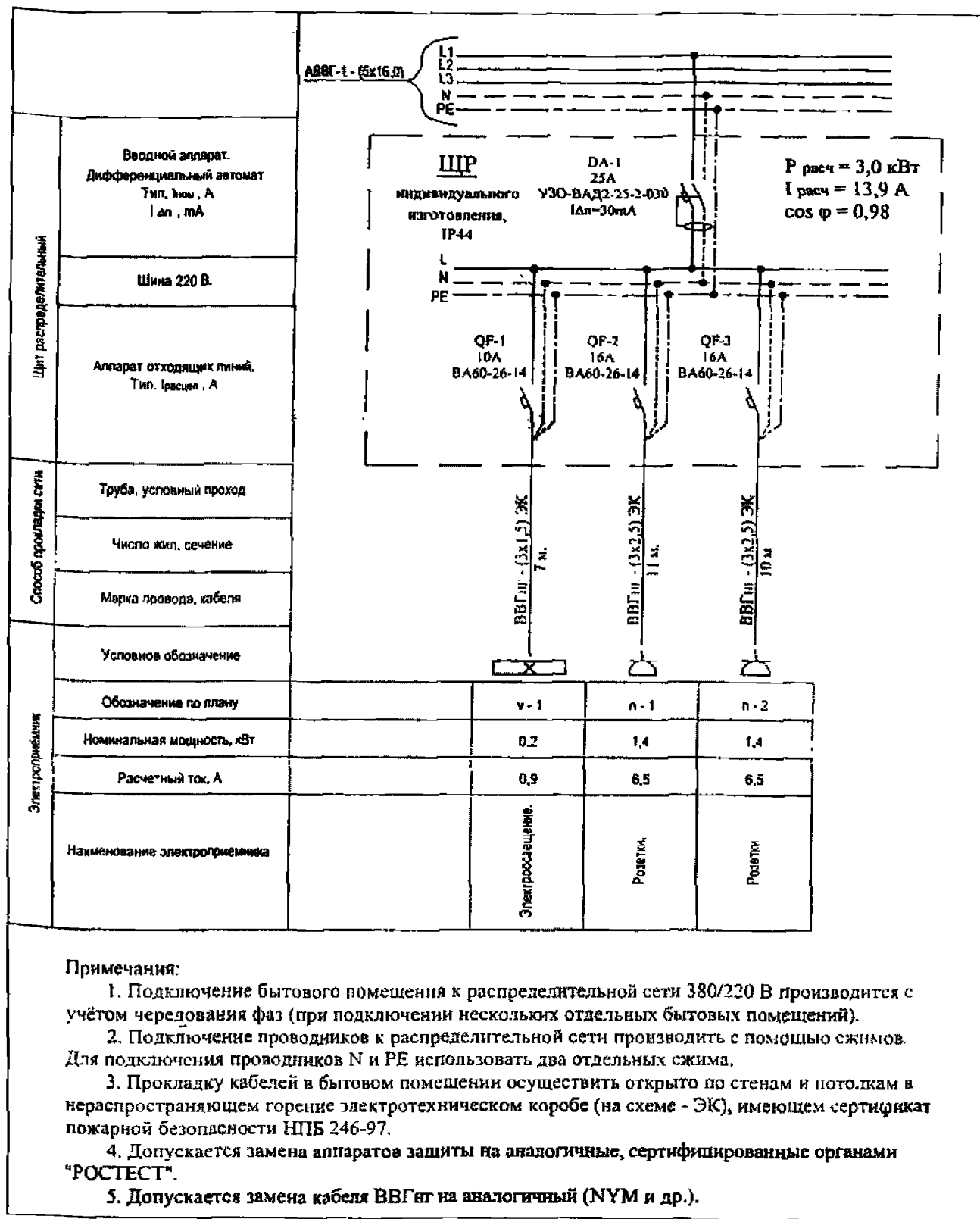
Рисунок 15 – Схема внутреннего электроснабжения бытового помещения
