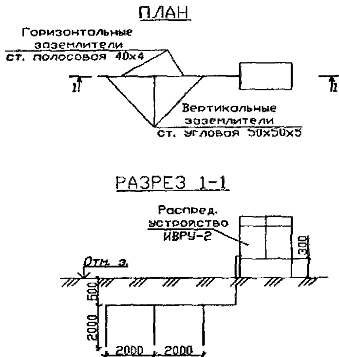
Рисунок 7 – Схема устройства заземления ИВРУ
