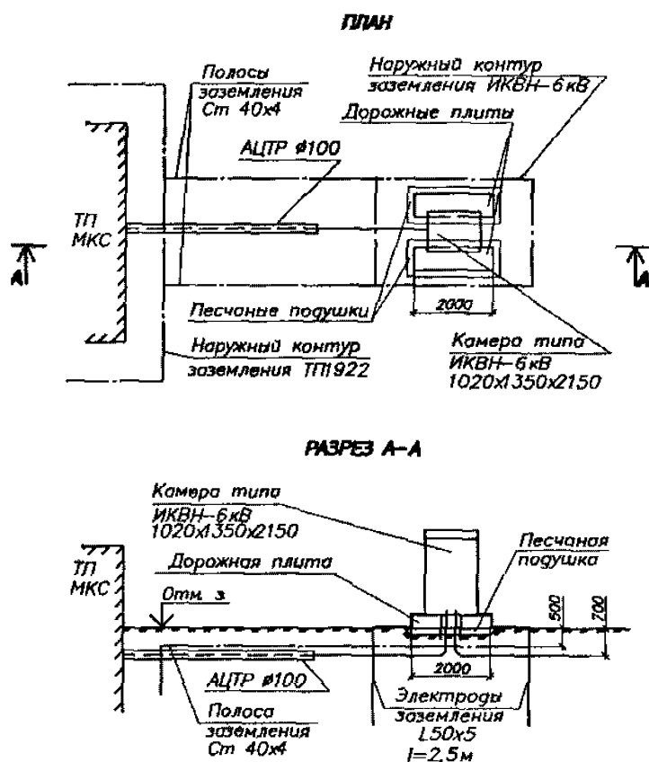
Рисунок 6 – Схема заземления ИКВН
