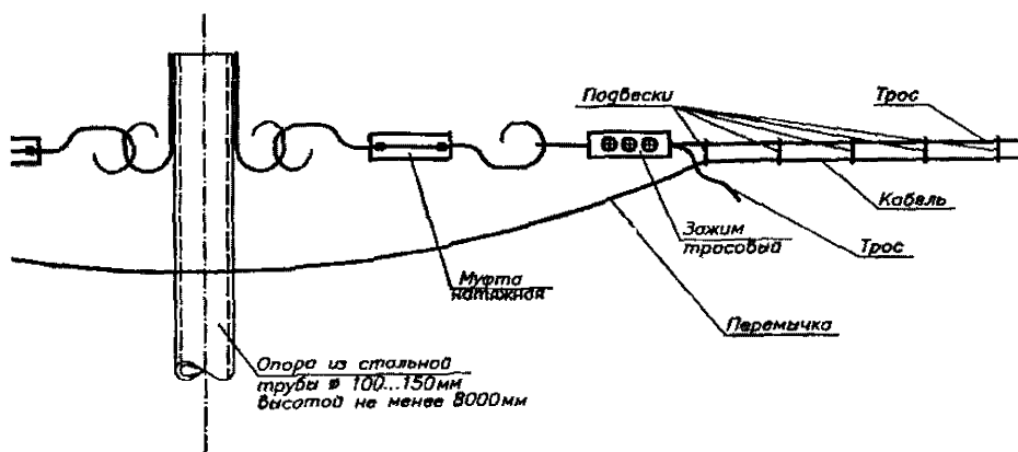
Рисунок 13 – Схема закрепления кабельных линий к временным опорам
