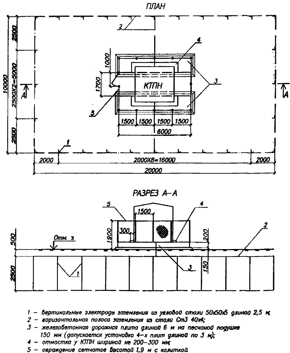
Рисунок 3 – Вариант временного ограждения КТПН
