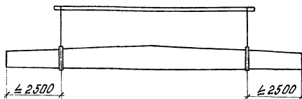
Рис.2 Строповка балок
