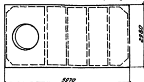
Плиты размером 3×6 м с отверстиями диаметром 1000 и 1450 мм (выпуск 1)
