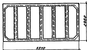
Плиты размером 3×6 м для легкосбрасываемой кровли (выпуск 2)
