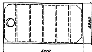
Плиты размером 3×6 м с отверстиями диаметром 400 и 700 мм (выпуск 1)
