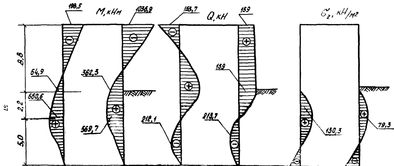
Рис. 16. Расчетные значения M_z , Q_z и \sigma_z по длине откола сваи.
