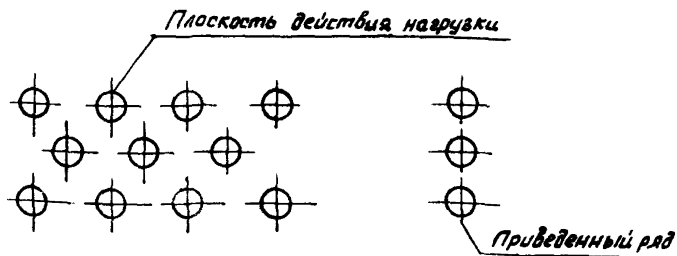
Рис. 6. Схема к определению условной ширины свай, B_c , при шахматном их расположении.
