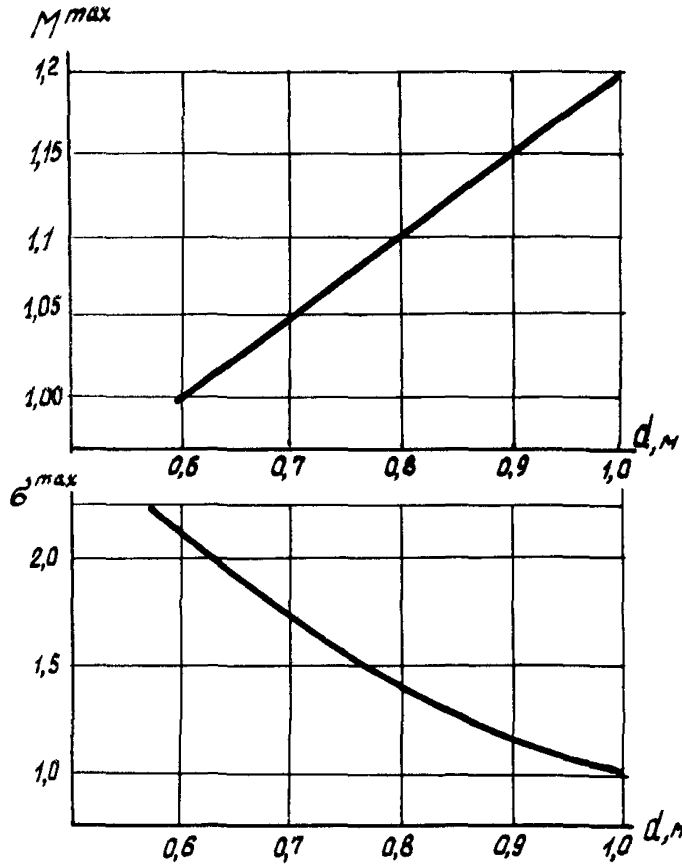
Графики изменения расчетных величин M , \sigma и \gamma_0 в зависимости от диаметра свая, d .
