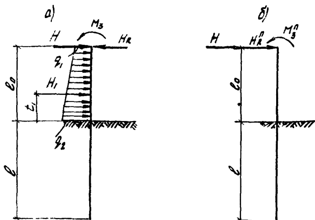
Рис. 5. Схема нагрузок для определения при многорядном расположении свай Q_x , M_x и Q_z .
