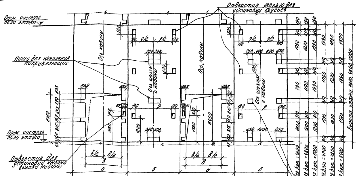
Вид по стрелке "А" по стрелке "А" бруска 130x180
