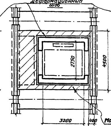
Грузовой лифт Q=2000кгс Q=3200кгс Кабина 2000 x 3000 x 2200
