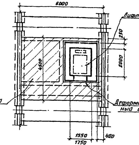
Лифт пассажирский Q = 500 кг Кабина 1080 × 1420 × 2100 и 1200 × 1400 × 2100
