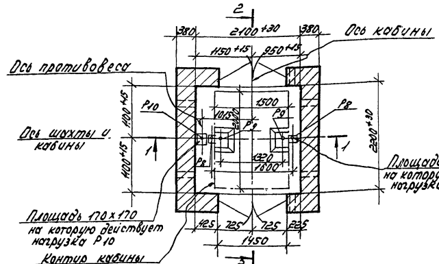
План шахты Вариант I
