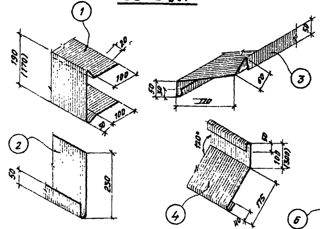
Узел А
