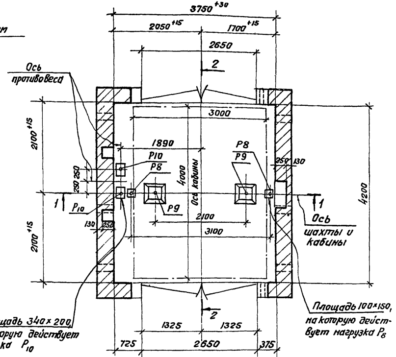
План шахты
