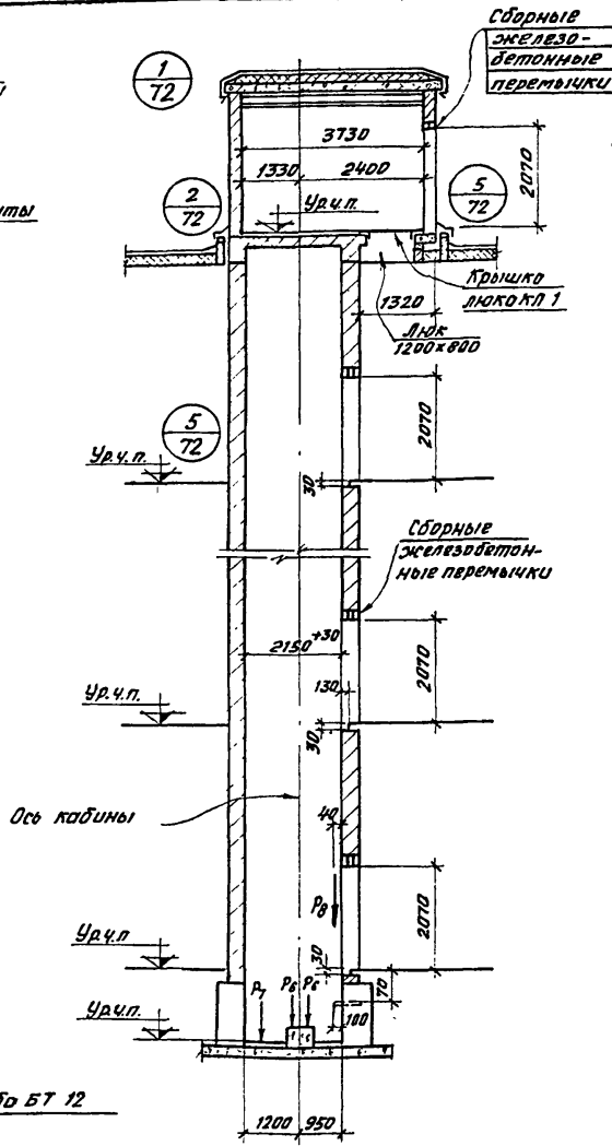
Разрез 2-2
