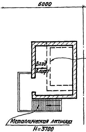
Лифт грузопассажирский Q=500кгс План машинного помещения
