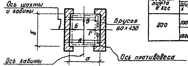
Схематический план шахты (Вариант II)
