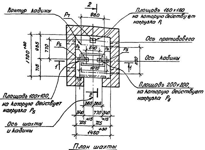
План шахты
