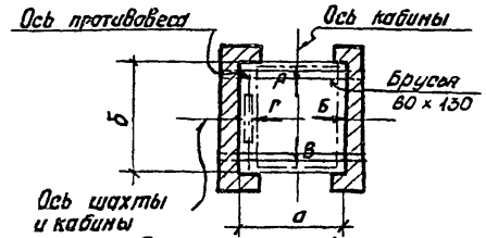
Схематический план шахты (Вариант I)
