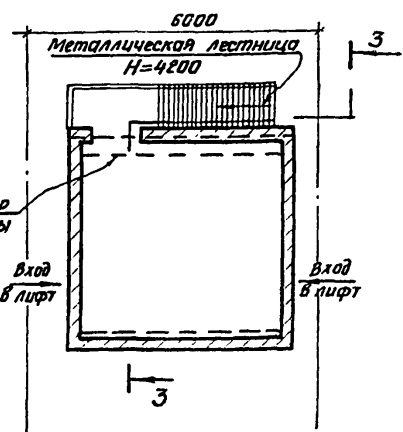
Лифт грузовой Q=500кгс План машинного помещения
