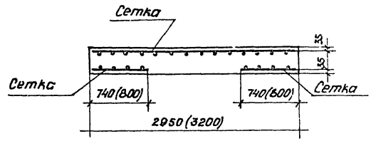
Армирование фундаментной плиты
