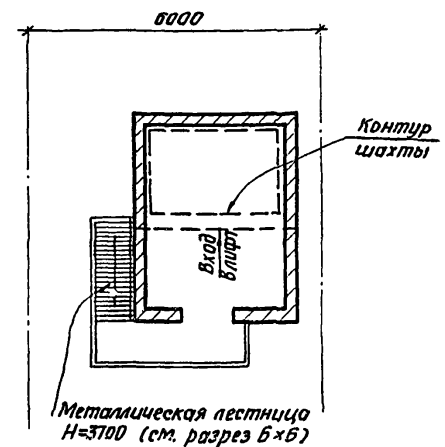
Лифт пассажирский Q=500кгс Кабина 2,2x1,2x2,1 План машинного помещения
