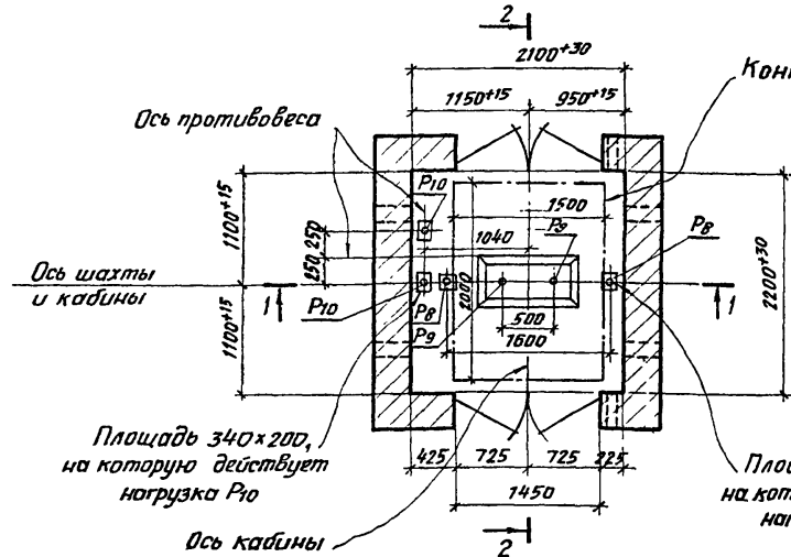
План шахты Вариант I
