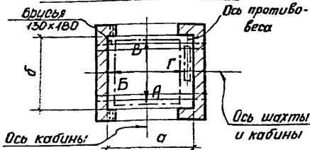
Схематический план шахты (Вариант II)
