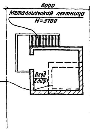
Лифты пассажирские Q=500кг, Q=350кгс и 320кгс План машинного помещения
