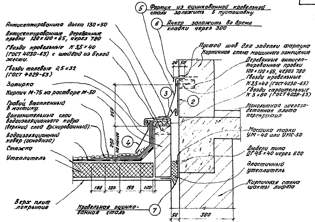
Узел Б
