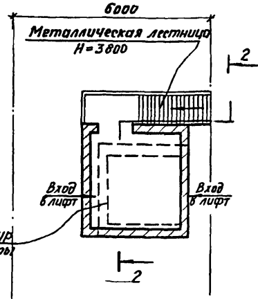
Лифт грузовой Q=1000кгс План машинного помещения
