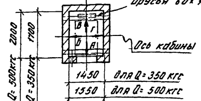
Схематический план шахты.
