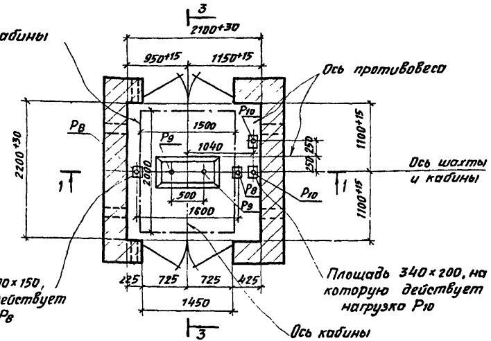
План шахты Вариант II
