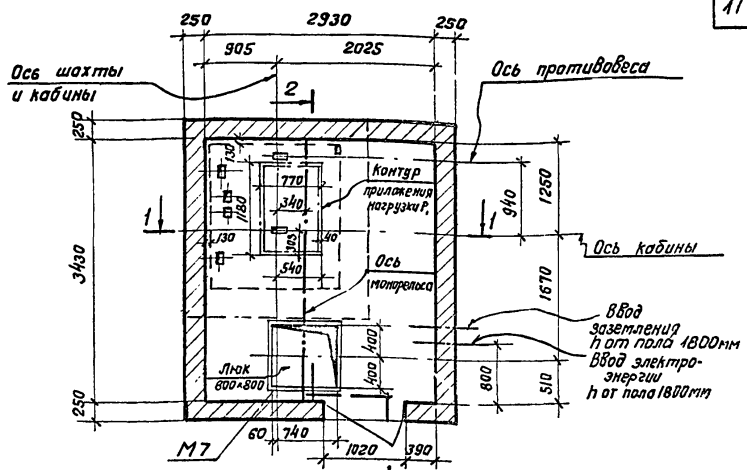
План машинного помещения Вариант II
