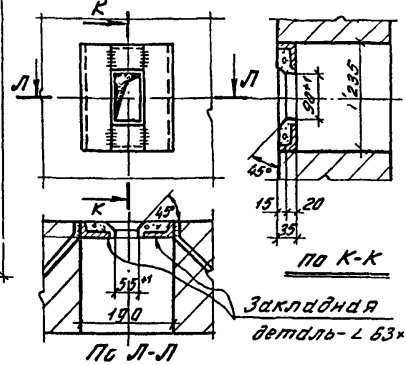
Деталь отверстия для установки кнопки вызова кабины для лифта Q = 350 кгс
