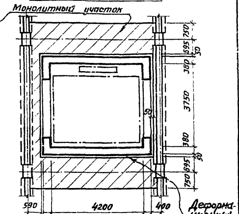
Грузовой лифт Q=5000кгс Кабина 3000 x 4000 x 2400
