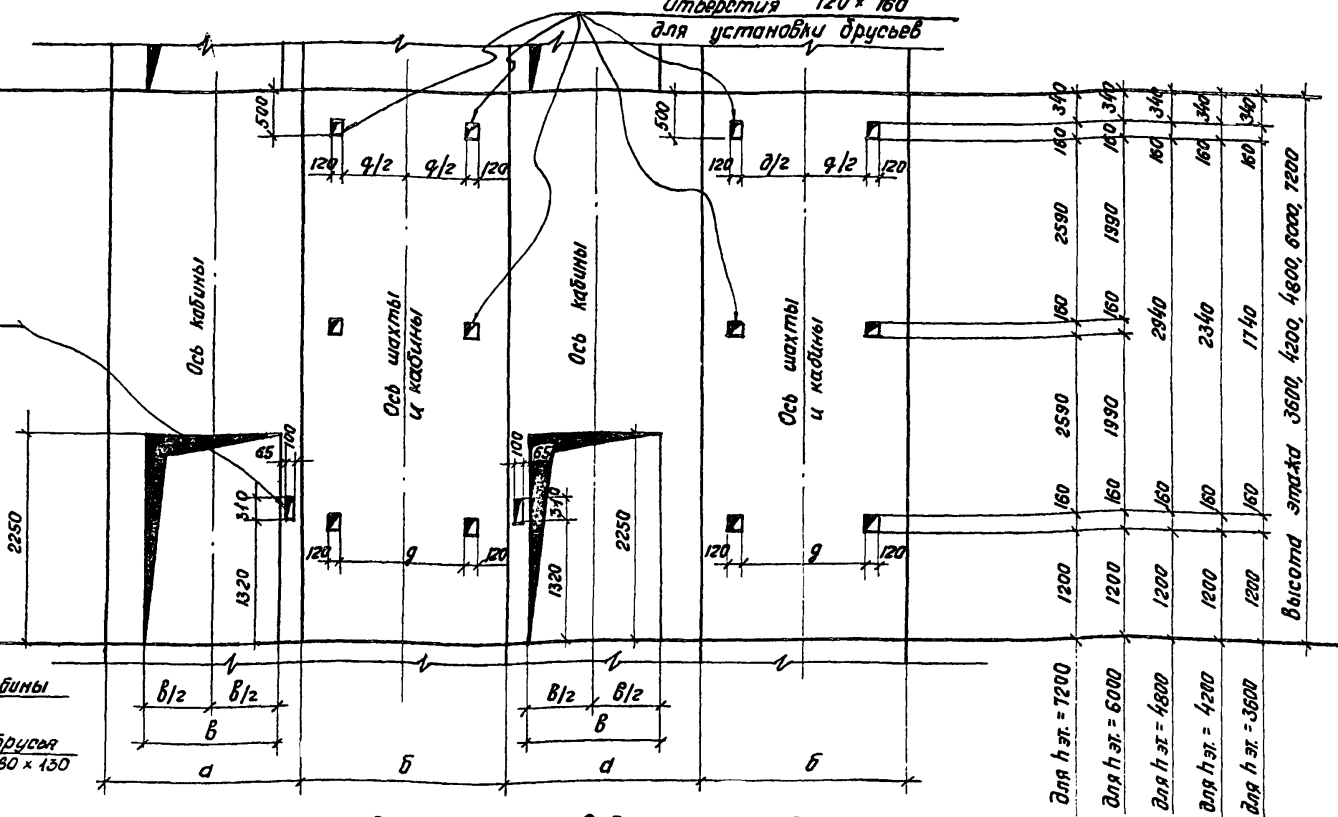
Вид по стрелке А, Вид по стрелке Б, Вид по стрелке В, Вид по стрелке Г
