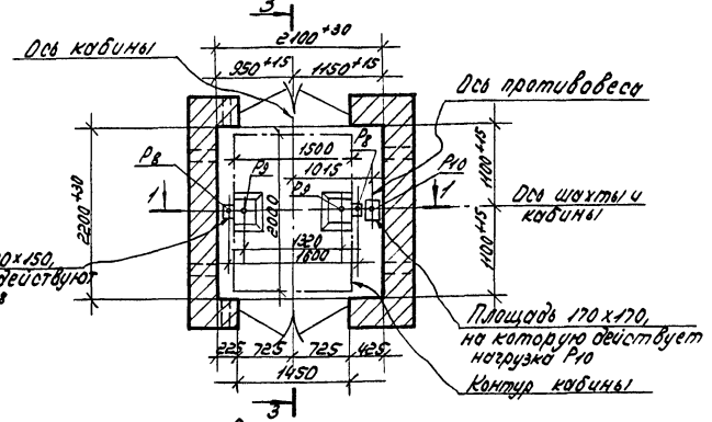
План шахты Вариант II
