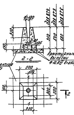
Бетонные тумбы БТ4, БТ5, БТ6
