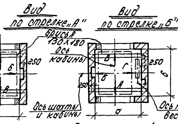
Схематический план шахты (вариант 1)
