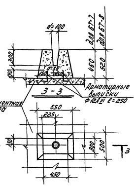
Бетонные тумбы БТ7, БТ8
