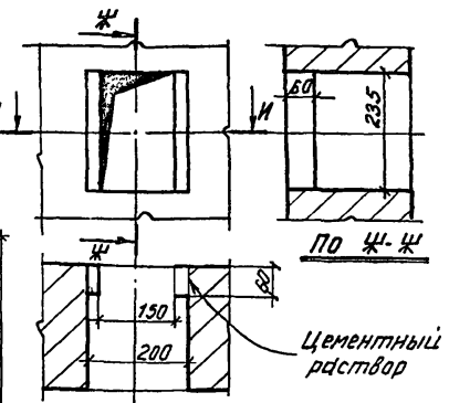
Деталь отверстия для установки кнопки вызова кабины для лифта Q = 500 кгс
