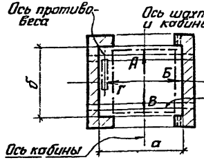
Схематический план шахты (Вариант I)
