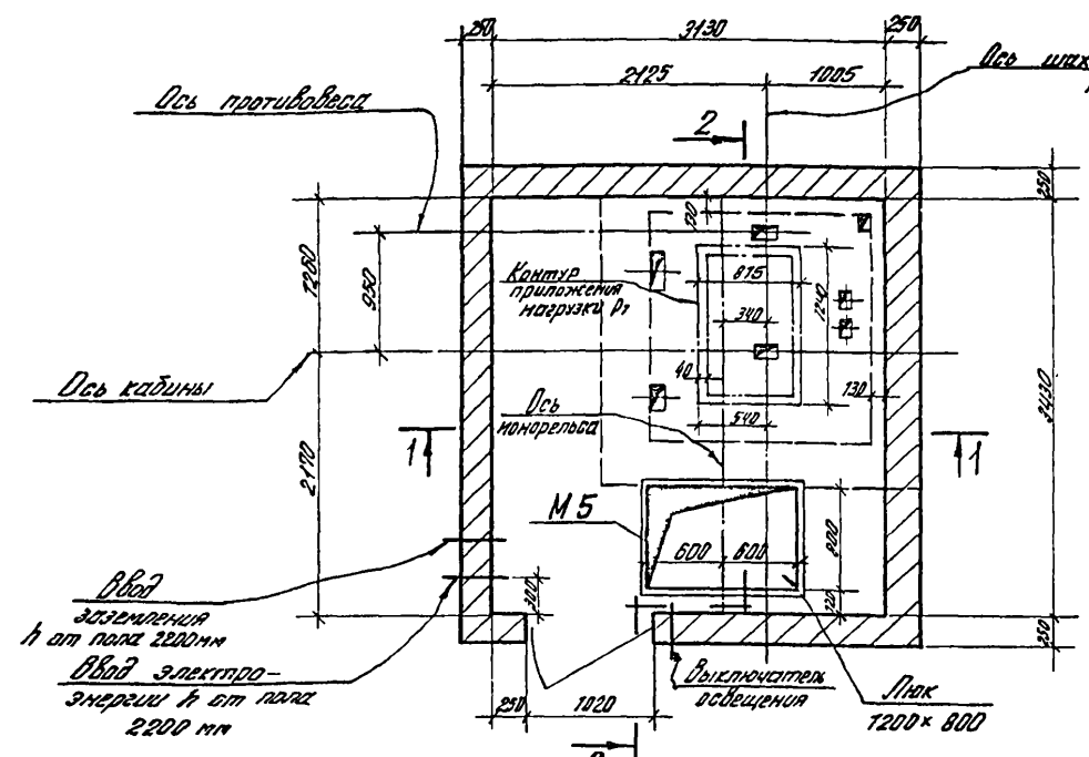
План машинного помещения Вариант I
