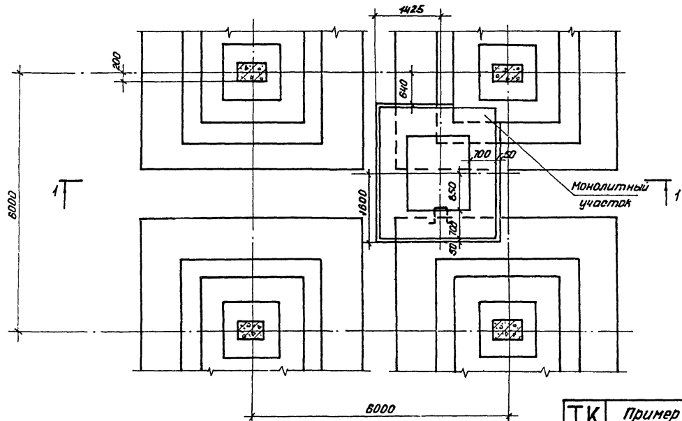
Армирование фундаментной плиты
