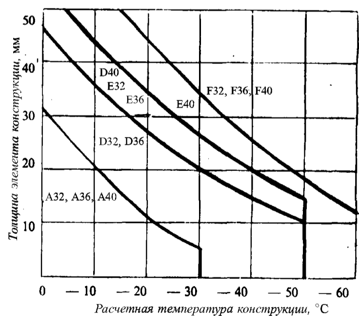
Рис. 1.2.3.1-3 Группа связей III
