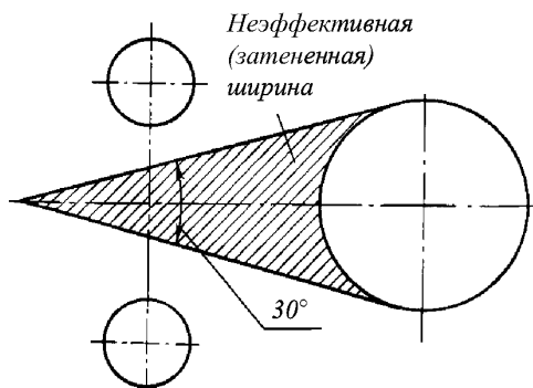
Рис. 1.4.8.3 Расчетное сечение
