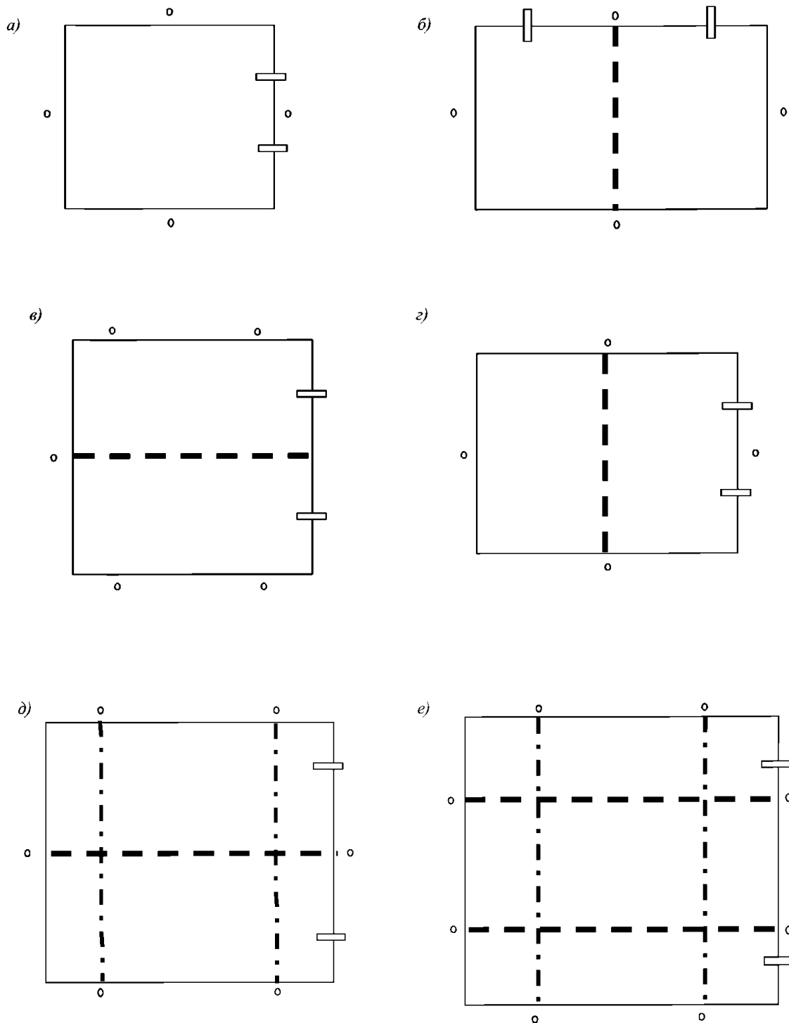
Рис. 7.7.2.2 Номинальные размеры люковых закрытий:
