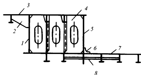
Рис. 2.12.5.6.6: 1 — опорная переборка; 2, 6 — кницы; 3 — квартердек; 4 — диафрагма; 5 — переборка уступа; 7 — верхняя палуба; 8 — ребро в плоскости кницы
