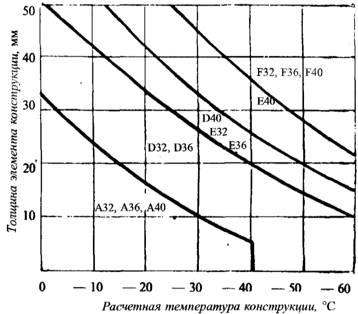
Рис. 1.2.3.1-2 Группа связей II
