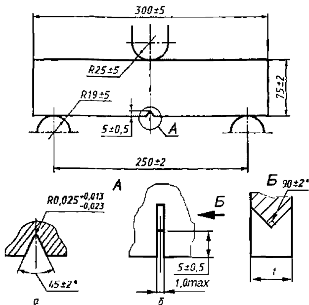
Рис. 1.2 Образец и оснастка для испытаний ( t – толщина)
