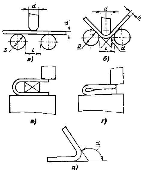
Рис. 3.1 Схема испытаний на изгиб
