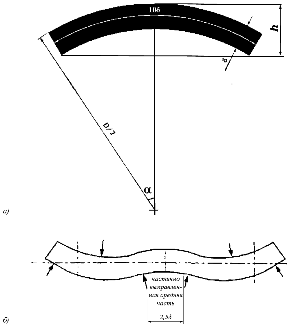
Рис. 2.1 Правка поперечных заготовок из трубы
