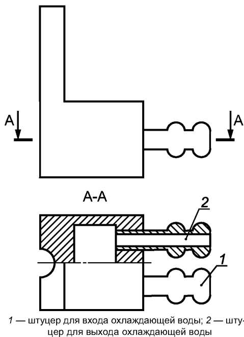
Рисунок 4 — Электрододержатели
