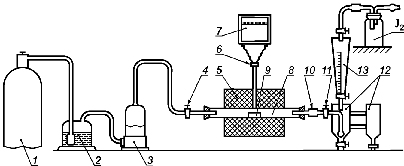
1 — баллон с кислородом, снабженный редукционным вентилем для регулирования скорости поступления кислорода в печь; 2 — промывная склянка, содержащая раствор марганцовокислого калия в растворе гидроксида калия или гидроксида натрия; 3 — склянка, содержащая в нижней части плавленный хлористый кальций и слой стеклянной или обыкновенной ваты, а в верхней части — гидроксид калия или гидроксид натрия; 4 — кран, дающий возможность регулировать подачу очищенного кислорода в трубки для сжигания; 5 — трубчатая печь с силитовыми нагревателями, обеспечивающими нагрев до 1250 °С; 6 — термопара; 7 — милливольтметр или потенциометр любого типа; 8 — трубки для сжигания кислорода; 9 — лодочка для сжигания пробы; 10 — очистительный сосуд с кварцевой ватой; 11 — кран перед поглотительным сосудом; 12 — поглотительный сосуд, состоящий из двух одинаковых сосудов, соединенных стеклянными перемычками. Допускается использование двух стеклянных цилиндров высотой по 250 мм из стекла одного цвета (рисунок 2); 13 — бюретка для титрования
