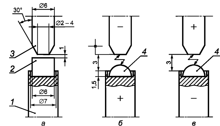
а — расположение электродов и брикета до экспонирования; б — съемка в анодном режиме; в — съемка в катодном режиме 1 — графитовая подставка; 2 — брикет; 3 — подставной электрод; 4 — расплав
