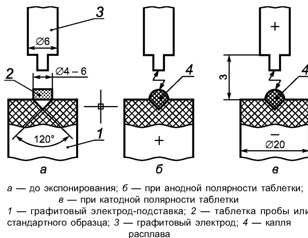
Рисунок 5 — Графитовые электроды
