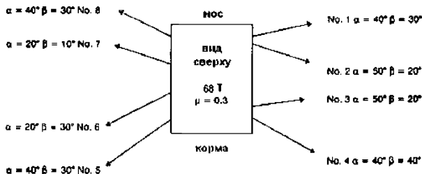
Рис. 5 Общий вид грузового места, раскрепленного 8-ю найтовыми
