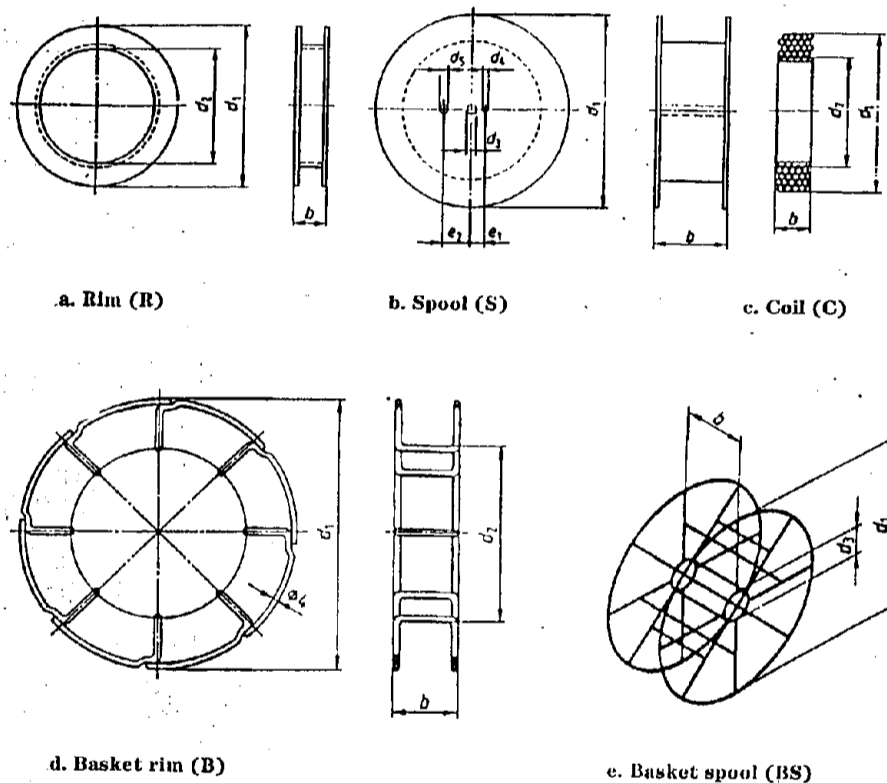
Рис. 5.3.3.3.3 Виды намотки сварочной проволоки для поставки потребителям: a — кольцевая обойма (R); b — катушка (S); c — моток квадратного сечения (C); d — корзинчатая кольцевая обойма (B); e — корзинчатая катушка (BS)
