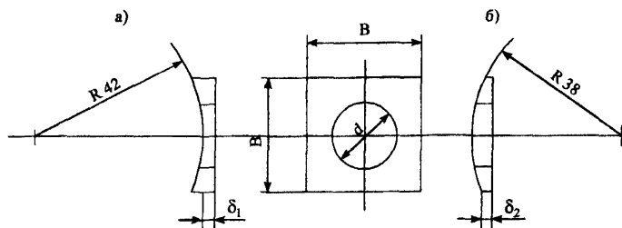
Рис. Б.1. Шайбы для болтов (размеры в миллиметрах): а — плоскогогнутые; б — плосковыпуклые; d — диаметр отверстия в шайбе (согласно ГОСТ 11371-68*); B — размер квадратной шайбы, принимаемый равным наружному диаметру стандартной круглой шайбы (согласно ГОСТ 11371-78*); \delta_1 — не менее 3; \delta_2 — не менее 2
