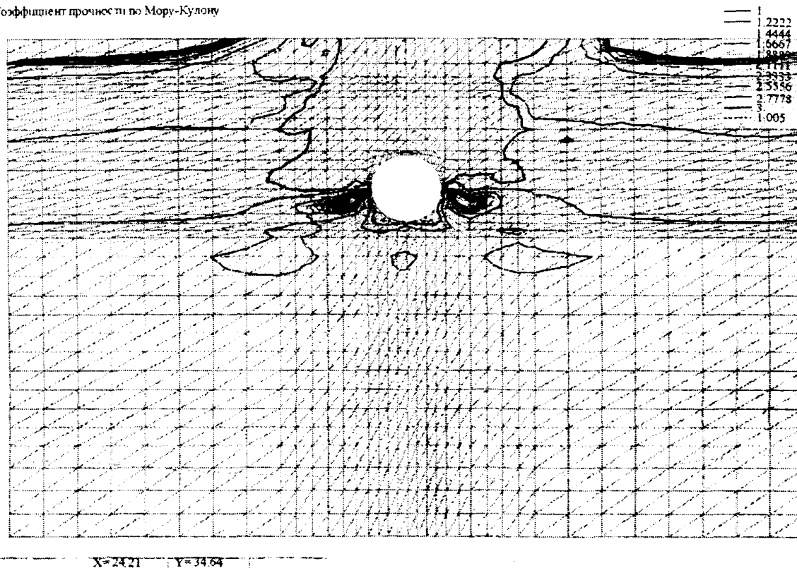
Рис. В.7. Коефіцієнт прочності по Мору-Кулону
