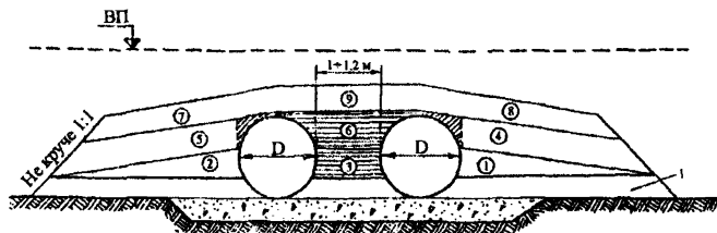
Рис. 27. Технологическая последовательность и схема послойного уплотнения грунта засыпки многоочковых МГТ:
