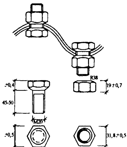
Тип М20,SB 8,8
