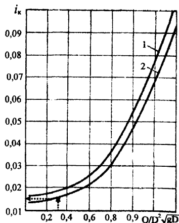
Рис. 5.27. График для определения критического уклона i_k для круглых гофрированных труб с гладкими лотками ( n_{лс} = 0,025 ): 1 – D=1,5 м; 2 – при D=2,0 м
