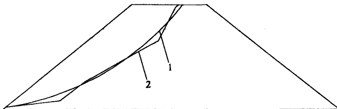
Рис. Ж. 4. Положение потенциальной кривой скольжения:
