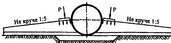
Рис. 22. Схема засыпки и уплотнения грунта наклонными слоями
