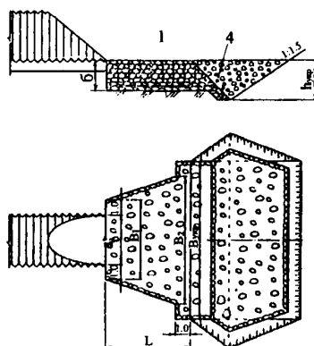
Рис. Е.4. Типы выходных русл из каменной наброски: а — тип I; б — тип II; в — тип III;
