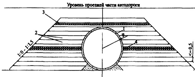
Рис. 10. Конструкция обоймы из армированного грунта: 1 – демпфирующий слой; 2 – слой армированного грунта, толщиной 0,5 м; 3 – слой объемной георешетки, распределяющий нагрузку; 4 – горизонтальные упоры из объемной георешетки
