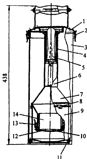
Рис. Л. 1. Схема плотномер-влажмера Н. П. Ковалева:
