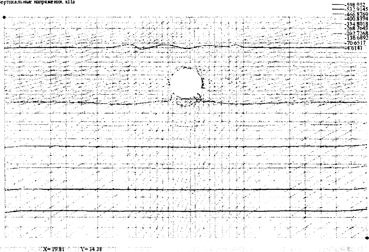
Рис. В.4. Вертикальные напряжения
