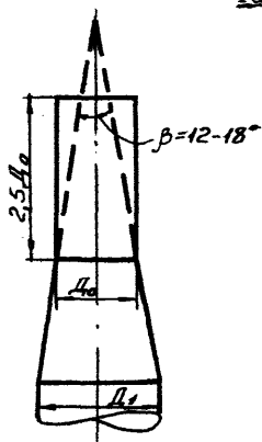
Эскиз факельного выброса
