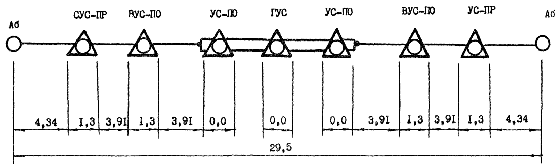
Рис.5.2. Распределение затухания,дБ,на ведомственной внутризоновой телефонной сети региона,бассейна (основной вариант)
