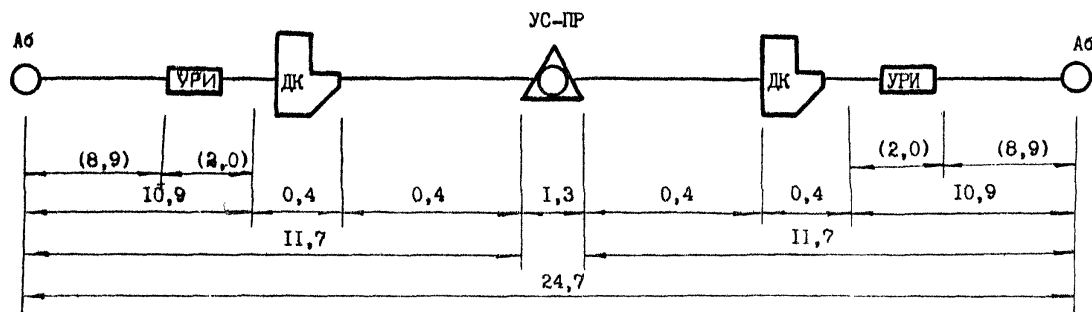
Рис.6.4.Распределение затухания,дБ,на телефонной сети предприятия (основной вариант)
