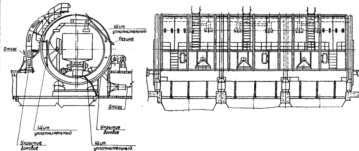
Укрытие роторного вагона генератора.
