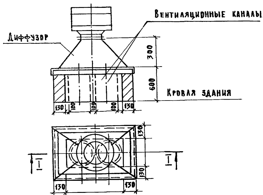
Рис. 7. Установка дефлектора на вытяжной шахте
