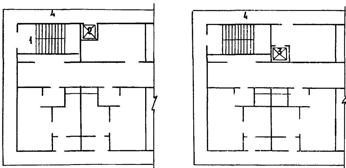
Рис. 3. Схемы размещения встроенных в здание лестницы и лифта, имеющих вход только с поэтажных галерей
