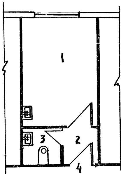
Рис. 6. Палата со шлюзом 1 — палата; 2 — шлюз; 3 — уборная; 4 — вход из коридора отделения
