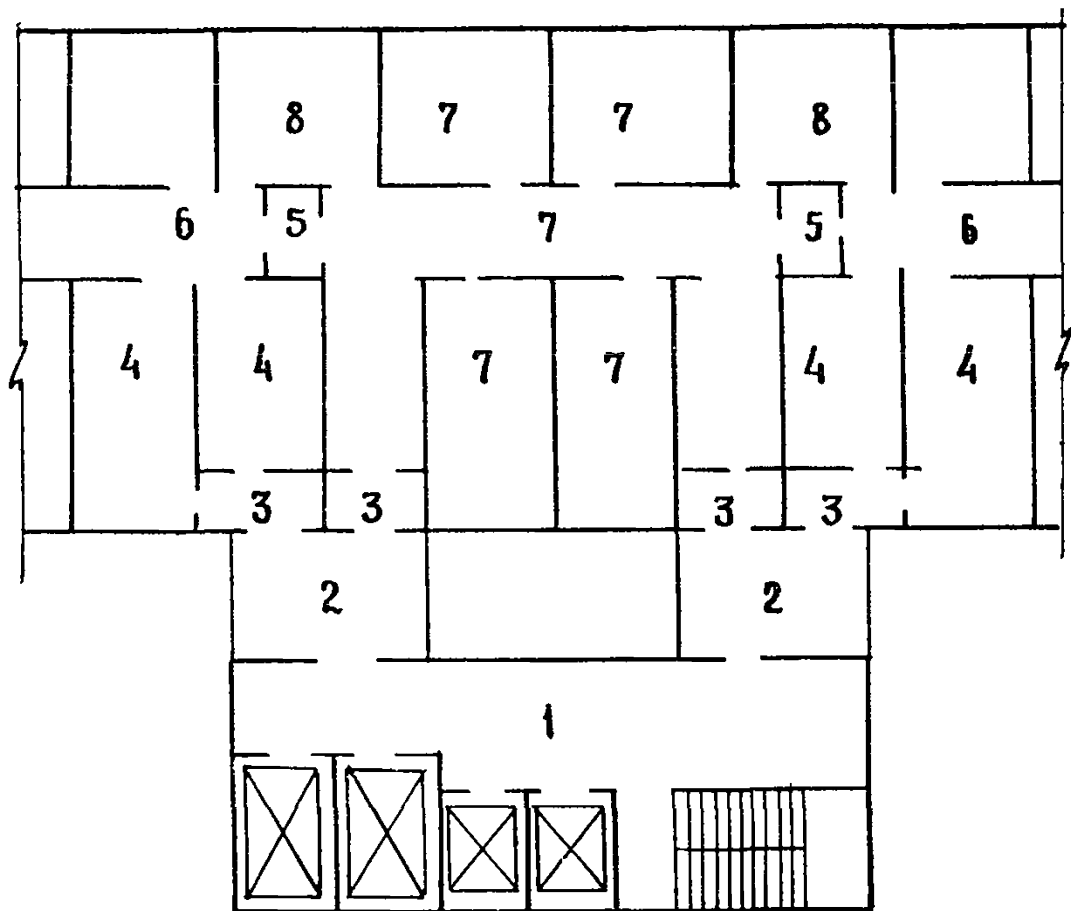
Рис. 2. Схема размещения выносного лестнично-лифтового узла для персонала (со стороны «чистой» зоны) с открытым переходом к зданию
