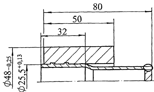
Рисунок 5 - Образец для испытаний на прочность
