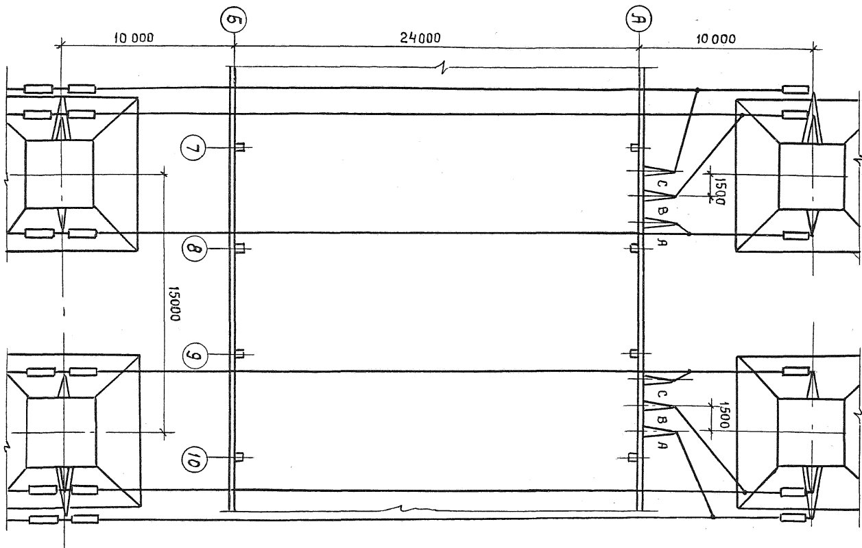
Пример перехода ошиновки над зданием ЗРУ. План (вариант с унифицированными анкерно-угловыми опорами типа УИО-I+4)
