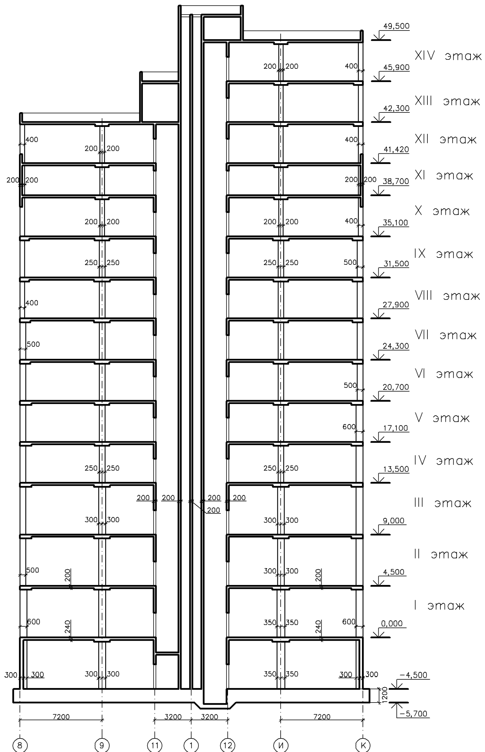
Рис.2. Разрез 1-1.
