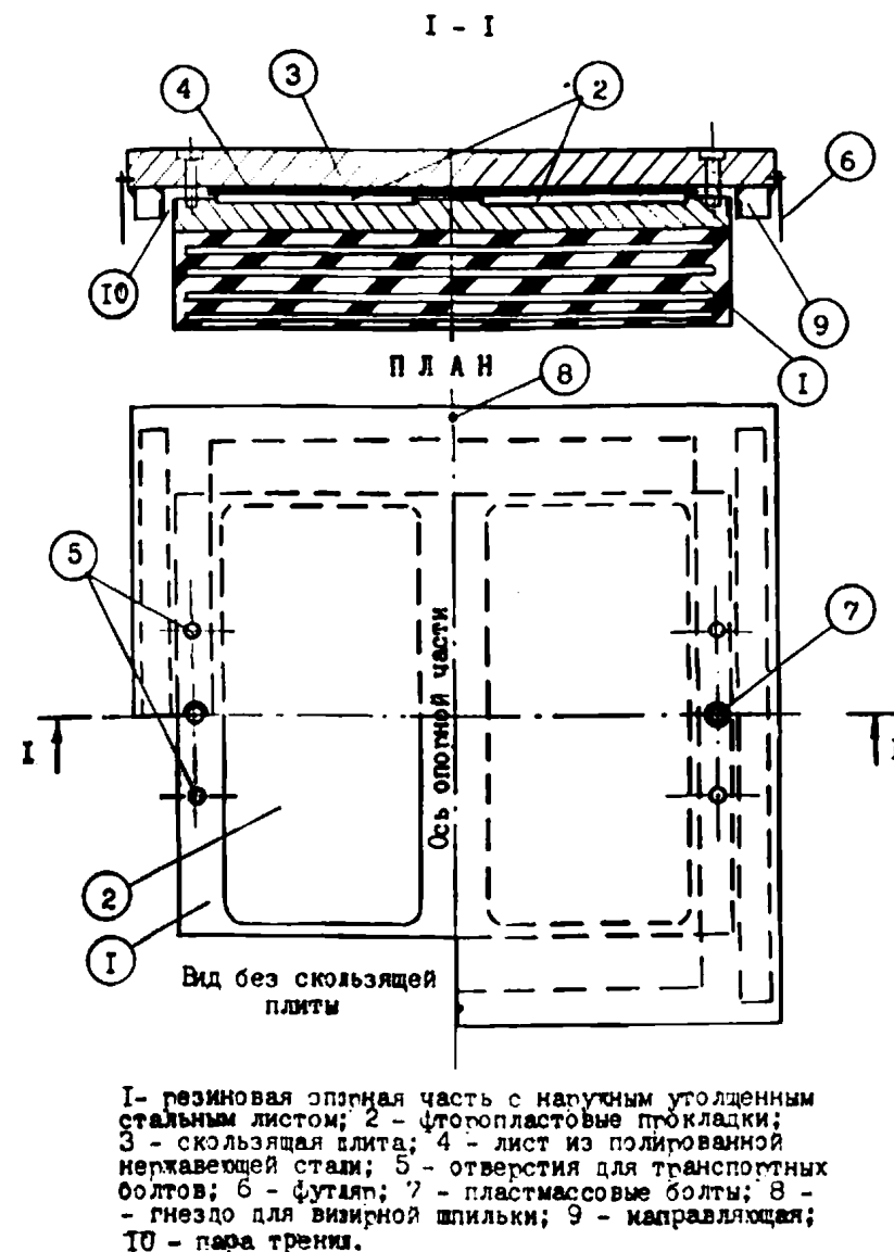
Рисунок 10. Конструкция линейно-подвижной резино-фторопластовой опорной части Л ДШР-РФОЧ (Тип 2)
