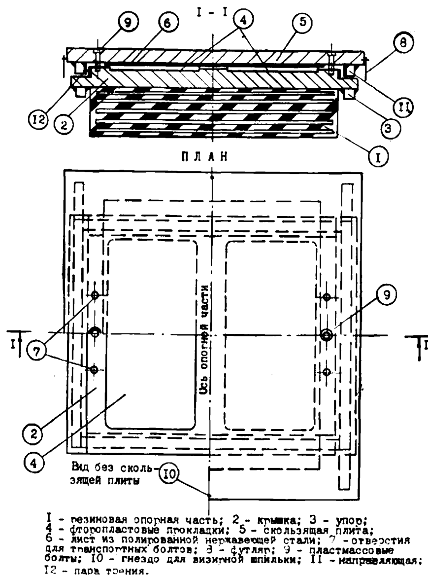
Рисунок 9. Конструкция линейно-подвижной резино-фторопластовой опорной части Л ДШР-РФОЧ (Тип 1)
