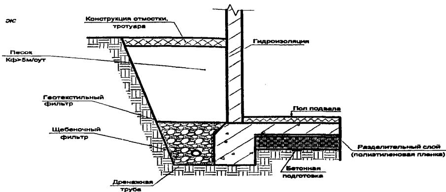
ж — с геотекстильной прослойкой в обсыпке дрена без геокомпозита
