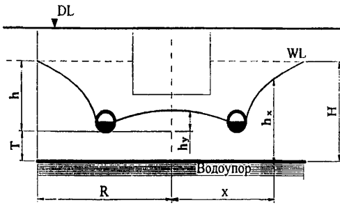
Рис. 11. Расчетные схемы контурного (кольцевого, пристенного) дренажа: а – совершенного типа; б – несовершенного
