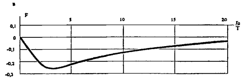
Рис. 13. Графики определения расчетных функций: а – \varphi_1 ; б – \varphi_2 ; в – F
