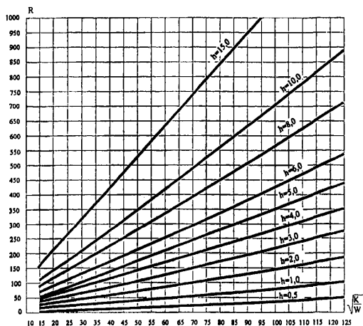
Рис. 10. График определения радиусов депрессии линейных dren
