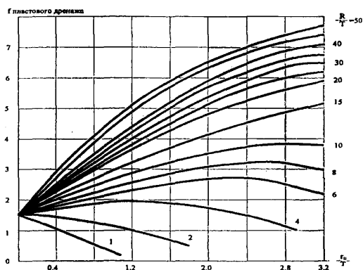
Рис. 16. График определения величины гидравлического сопротивления пластового дренажа
