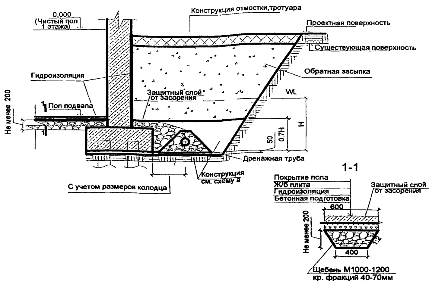
в – совершенного типа на условном водоупоре с линейным пластовым дренажем
