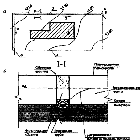
Рис. 2. Схема однолинейной системы дренажа совершенного типа:
