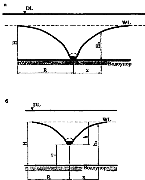
Рис. 9. Расчетные схемы однолинейного дренажа
