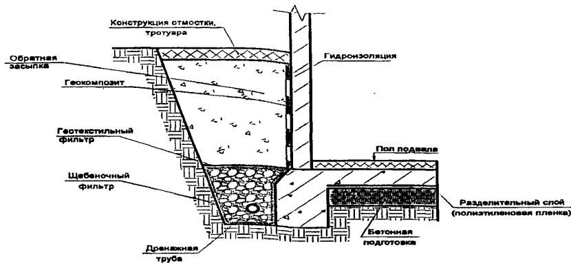
е — с геотекстильной прослойкой в обсыпке дрена и геокомпозитом
