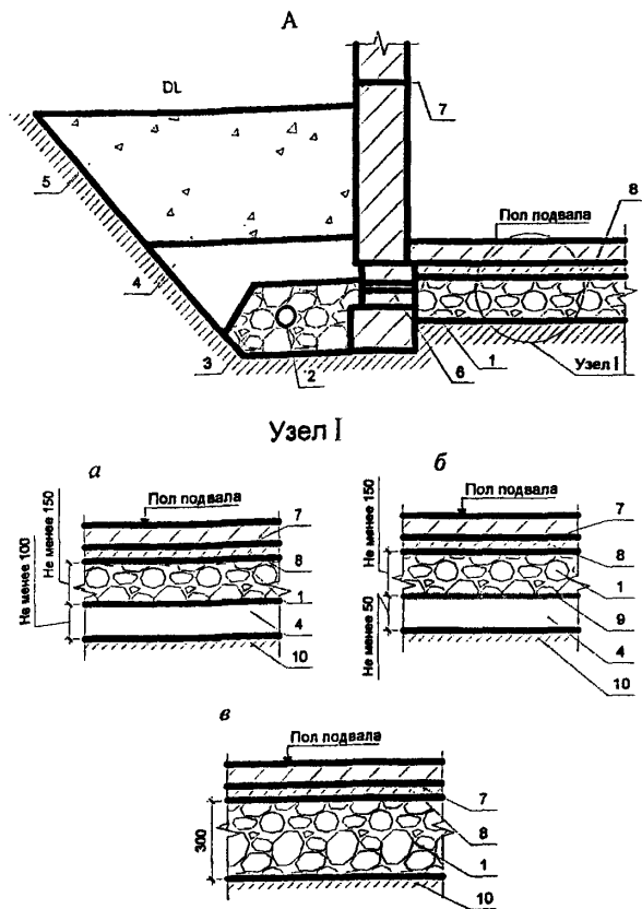
Рис. 7. Схема конструкции пластикового дренажа
