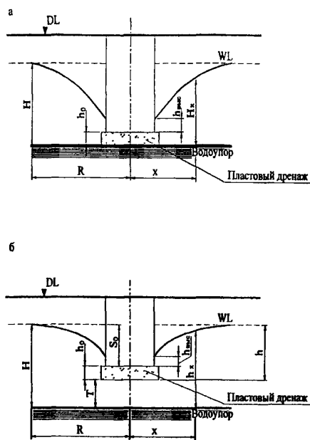
Рис. 15. Расчетные схемы пластового дренажа: а – совершенного типа; б – несовершенного
