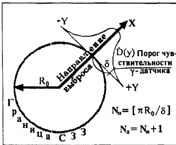
Рис. 1. Иллюстрация выбора оптимального количества датчиков АСКРО
