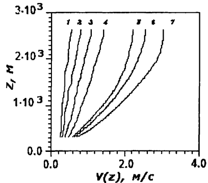
В Рис.3. Зависимость поперечной составляющей скорости ветра V(z) от высоты при различных состояниях устойчивости атмосферы (1-7) в модели пограничного слоя атмосферы
