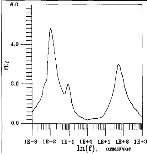
Рис.1. Спектр скорости ветра в приземном слое атмосферы [2].
