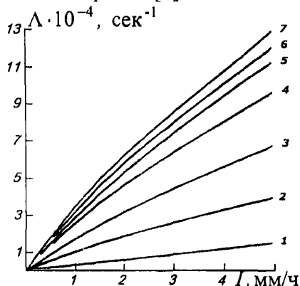
Рис.1 Коэффициенты вымывания частиц единичной плотности из подоблачного слоя атмосферы в зависимости от интенсивности дождя I для различных значений a^2 r (Chamberlain, 1953.) [4]: 1–4 \text{мкм}^2 \cdot \text{г}/\text{см}^3 ; 2–7,8 \text{мкм}^2 \cdot \text{г}/\text{см}^3 ; 3–16 \text{мкм}^2 \cdot \text{г}/\text{см}^3 ; 4–41 \text{мкм}^2 \cdot \text{г}/\text{см}^3 ; 5–81 \text{мкм}^2 \cdot \text{г}/\text{см}^3 ; 6–169 \text{мкм}^2 \cdot \text{г}/\text{см}^3 ; 7–400 \text{мкм}^2 \cdot \text{г}/\text{см}^3 .
