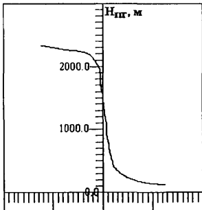
Рис. 1. Зависимость высоты пограничного слоя атмосферы от состояния ее устойчивости, характеризуемой параметром \mu_0 .
