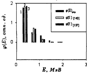
Рис.1. Гистограммы спектров фотонного излучения: 1 – исходный \phi(E)_{\text{исп}} ( E_{\text{сп}}=0,567 МэВ), 2 – восстановленный с использованием метода Y. Su ( E_{\text{сп}}=0,526 МэВ), 3 – восстановленный с использованием метода регуляризации Тихонова А.Н. ( E_{\text{сп}}=0,512 МэВ)
