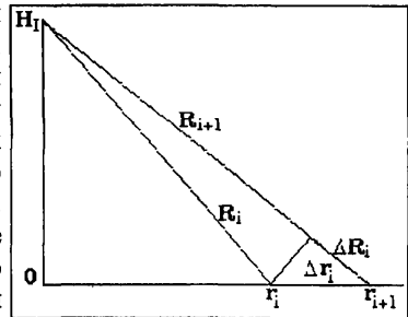
Рис.3. Определение приращения радиус-вектора R_i и его последующего значения по предыдущему. H_i - высота источника; r_i - расстояние на подстилающей поверхности от основания источника до детектора фотонного излучения АСКРО
