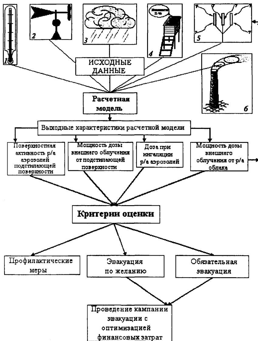
Рис.1 Структурная схема АСКРО: 1 – датчики температуры окружающей среды; 2 – датчики направления и скорости ветра; 3 – датчики осадков; 4 – датчики влажности окружающей среды; 5 – датчики фотонного излучения постов контроля; 6 - технологические датчики параметров выброса радиоактивной примеси в атмосферу
