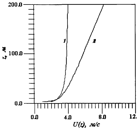
Рис.1. Зависимость скорости приземного ветра U(z) от высоты от подстилающей поверхности (модель приземного слоя атмосферы): 1 - неустойчивое состояние ( L=-18 , v_* = 0,32 м/с), 2 - устойчивое состояние ( L=30 , v_* = 0,26 м/с)
