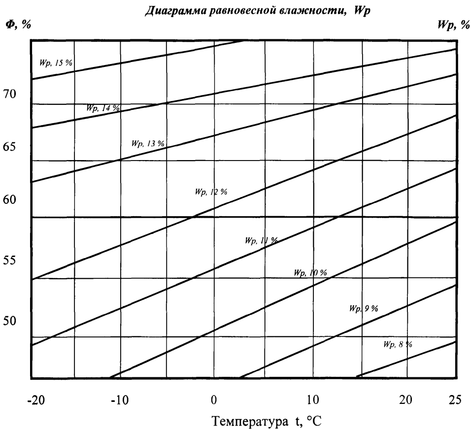
Рисунок 2 - Параметры режима хранения
