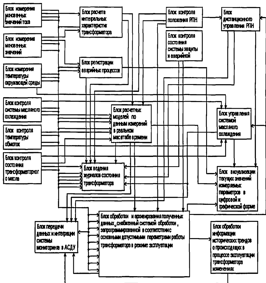
Рис. 2. Функциональная блок-схема.
