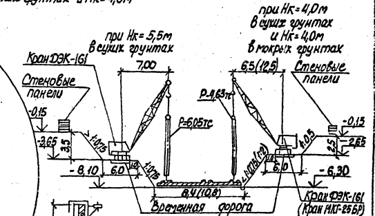
Разрез I-I
