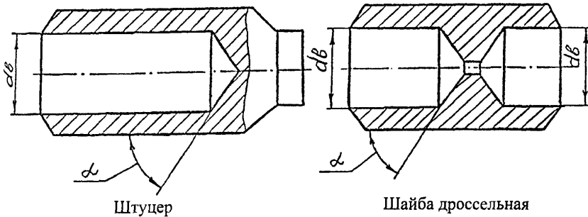
Штуцер
