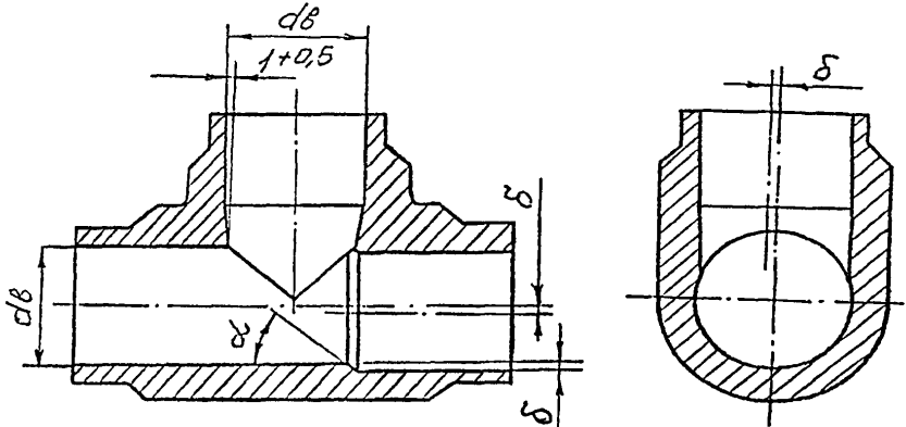
Тройник
