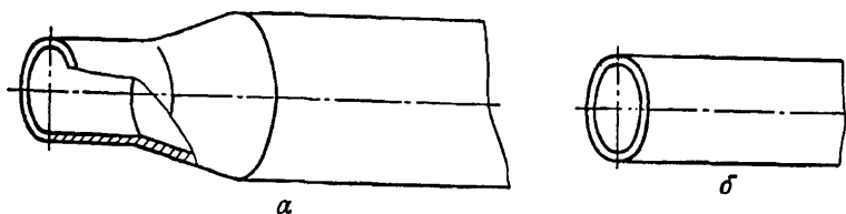
а- редуцированный конец трубы или перехода; б- торцы после калибровки Чертёж 27
