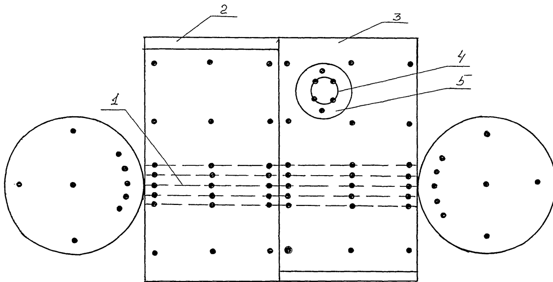
Схема измерения толщин элементов подземных резервуаров 1-нижняя образующая ; 2 и 3 - части обечайки 4- горловина люка ; 5- накладное укрепляющее кольцо .
