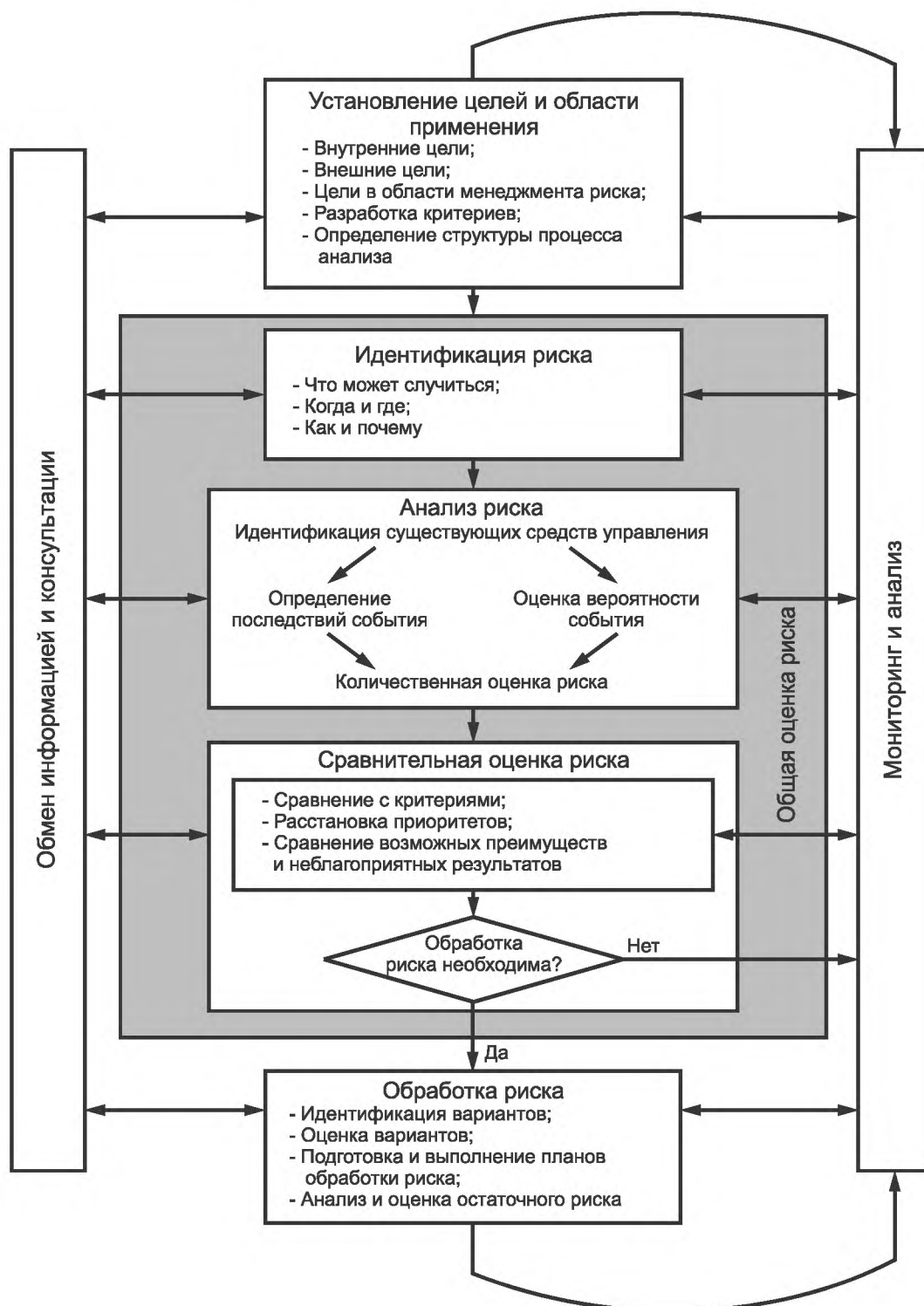
Рисунок А.1 — Подробное описание процесса менеджмента риска
