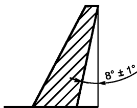
Рисунок 2 — Пирометрический контрольный конус с типичным углом наклона наружного ребра или грани
