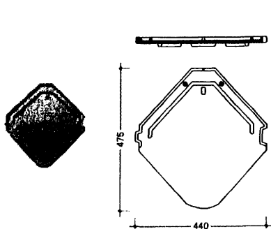
Рис. 19. План черепицы, поперечный и продольный разрезы.
