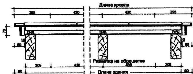
Рис. 21. Продольный разрез кровли с применением на фронтоне боковой черепицы (левой и правой).
