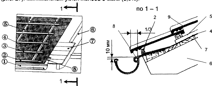
Рис. 27. Карнизный свес кровли.
