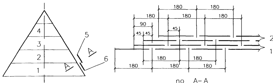
Рис. 29. Неравномерная укладка черепицы.
