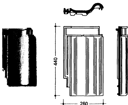
Рис. 7. План черепицы, поперечный и продольный разрезы.
