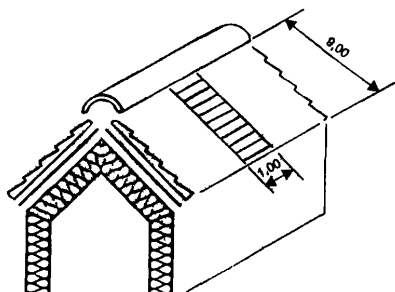
Рис. 25. К расчёту вентиляционного зазора на карнизном свесе.
