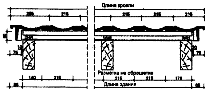
Рис. 15. Продольный разрез кровли с применением на фронтоне боковой черепицы (левой и правой)
