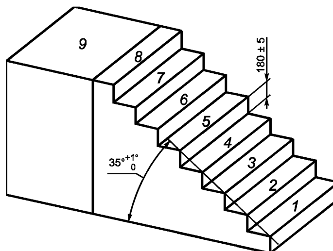
Рисунок 3 — Прямая испытательная лестница с верхней лестничной площадкой
