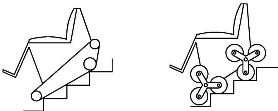
Рисунок А.5 — Типичный представитель самоустанавливающегося лестничехода с креслом, управляемого пользователем (тип Е)
