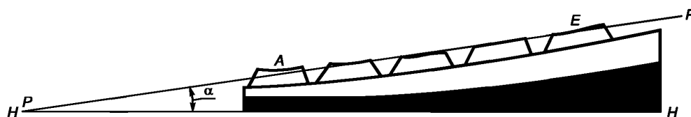
Рисунок 10 — Измерение наклона клавиатуры
