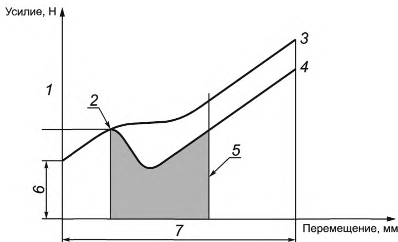
Удар по клавише и нажатие клавиши
