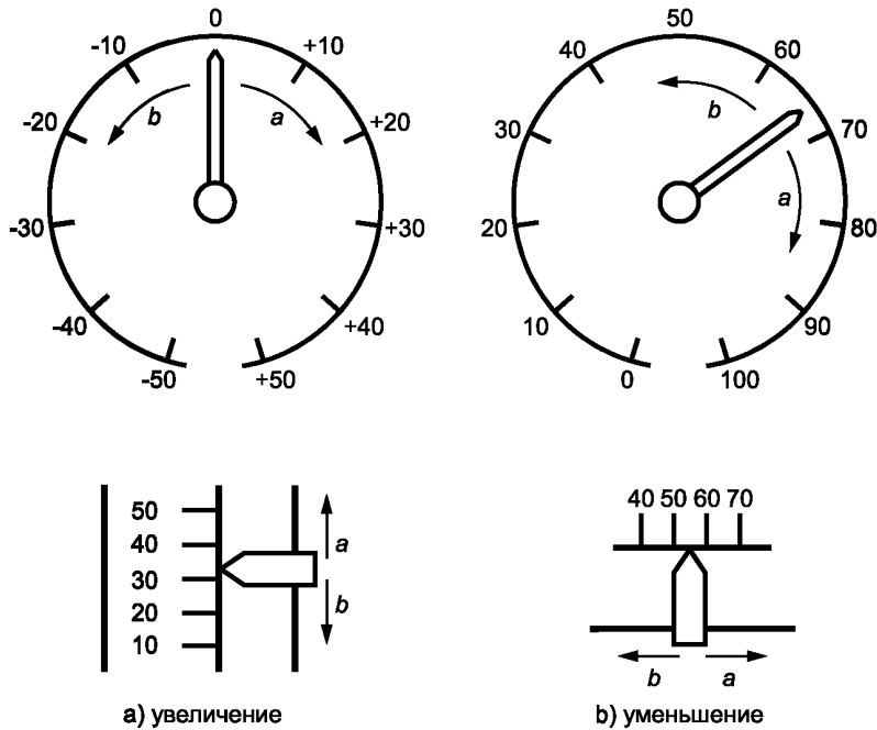
Рисунок 4 — Возможные направления перемещения указателя
