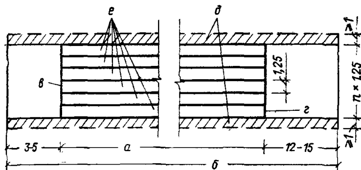
Рис. 8. План прямой беговой дорожки (размеры в м)
