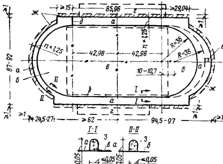
Рис. 9. План-схема спортивного ядра с полем для футбола и беговой дорожкой расчетной длиной 400 м (размеры в м)
