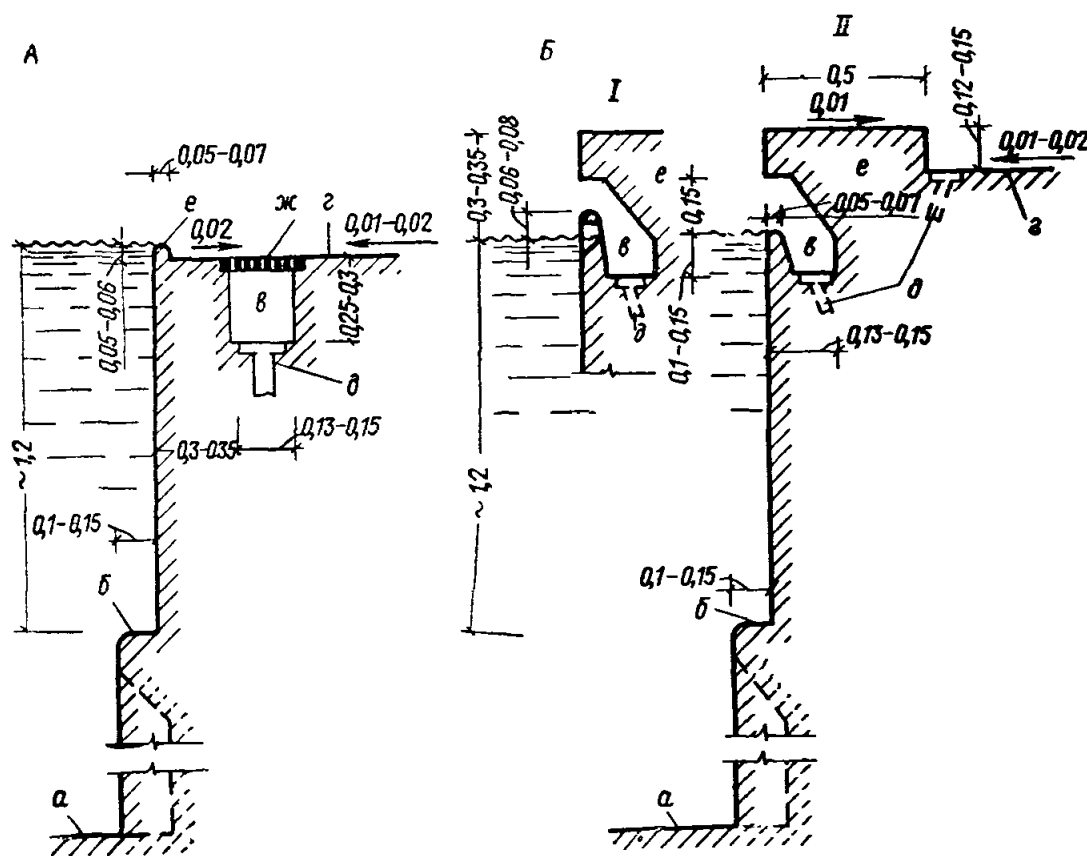
Рис. 12. Схемы профилей стенок ванн (размеры в м)
