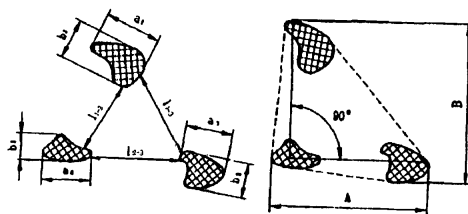
Рисунок А.40 Скопление включений
