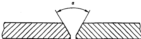
Рисунок А.18 Угол разделки кромок
