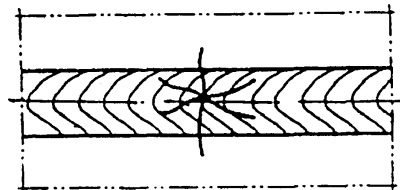
Рисунок А.27 Радиальные трещины сварного соединения
