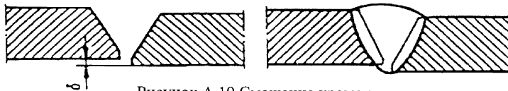
Рисунок А.19 Смещение кромок
