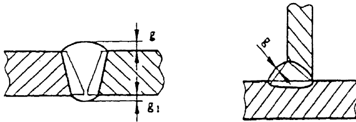
Рисунок А.9 Выпуклость сварного шва
