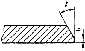
Рисунок А.17 Угол скоса кромки
