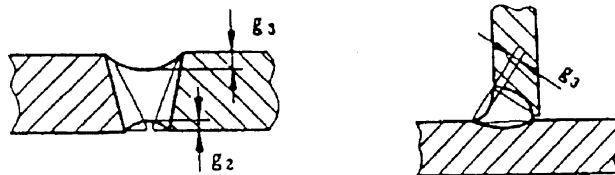
Рисунок А.10 Вогнутость сварного шва
