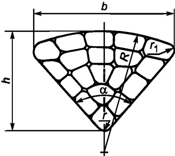
r_1 – радиус закругления, равный 1/2 диаметра проволоки
