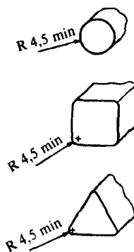
Рисунок Д.3 — Закругление краев элементов для крепления веревок (мм)
