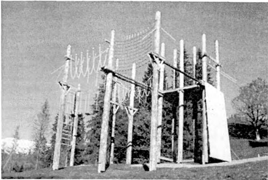
ПРИМЕР ПАРКА НА ДЕРЕВЯННЫХ СТОЛБАХ
