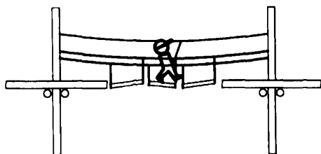
Змейка из висячих закрепленных бревен
