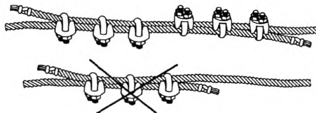
Рисунок В.4 — Размещение захватов проволоочного каната
