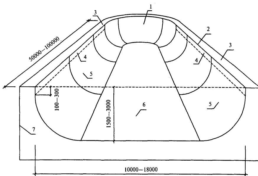
Б. ТРАДИЦИОННАЯ ТРУБА
