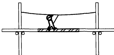
Переправа «Подвесной мост с разрывами» без перил
