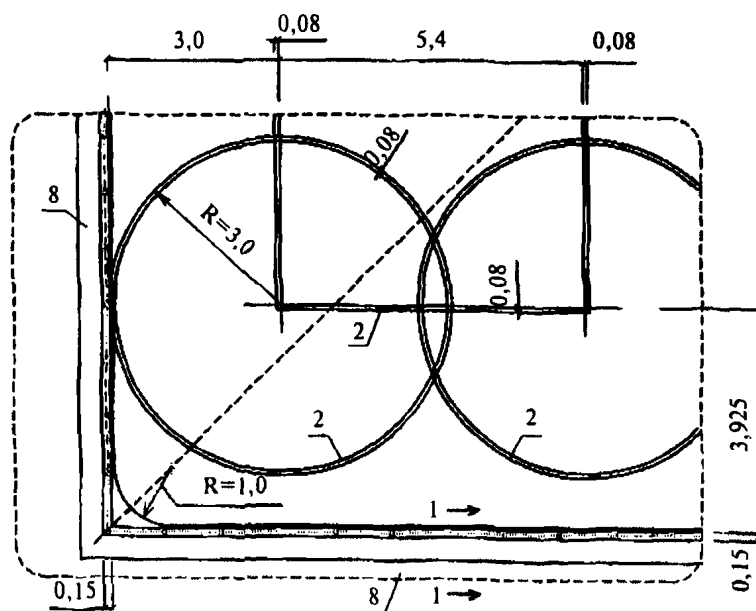
УЗЕЛ А
