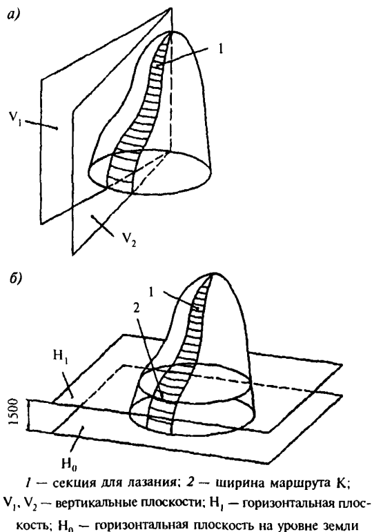
Рисунок Г.1 — Секция для лазания
