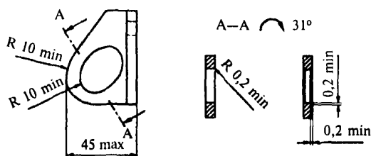
Рисунок Д.2 — Выступающая часть индивидуальной страховочной точки
