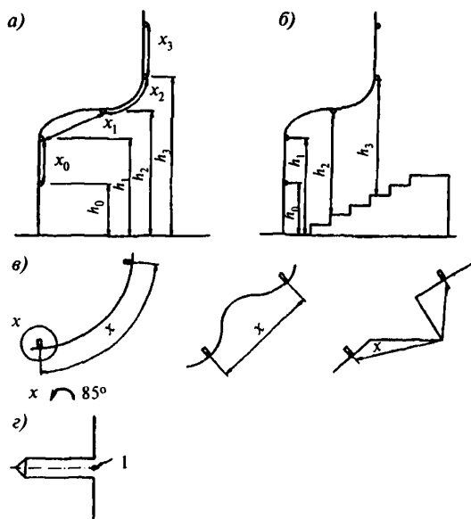
Рисунок Д.1 — Расположение и компоновка страховочных точек
