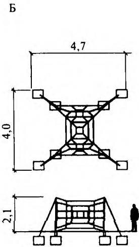
ПРИМЕРЫ ПРОСТРАНСТВЕННЫХ ПАРКОВ А — рации 3,5 — 16,4 — 7 Б — варио ВрК 2,1 — 4,7 — 4
