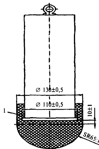
1 — силикон, размеры указаны в мм Суммарная масса (22 ± 0,1) кг
