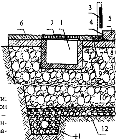
Б. ПРИМЕРЫ КОНСТРУКЦИЙ КРАЯ БЕГОВОЙ ДОРОЖКИ
