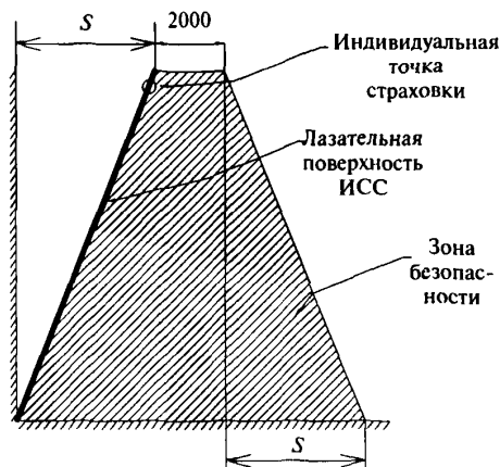
Схема 4.2 — Расчет зоны безопасности при использовании верхней страховки
