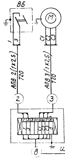
Схема подключения
