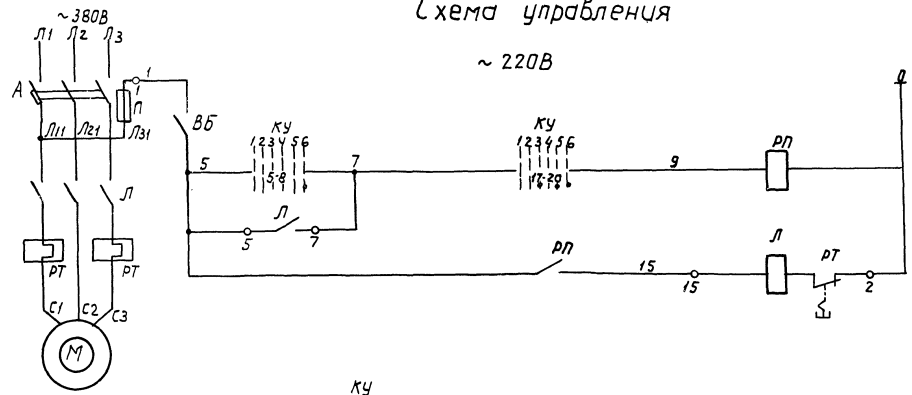
Схема управления
