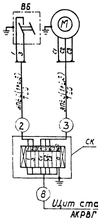
Схема подключения
