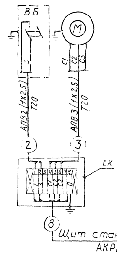
Схема подключения
