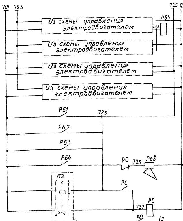
Из схемы технологической сигнализации
