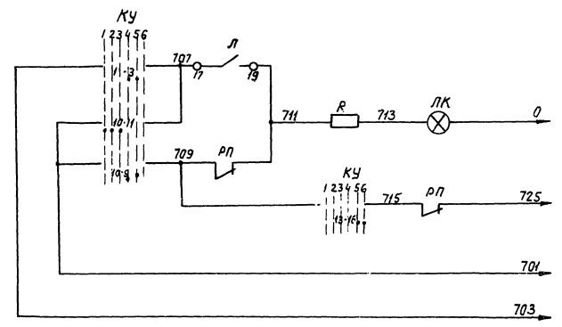
Диаграмму работы контактов КУ см. лист 2
