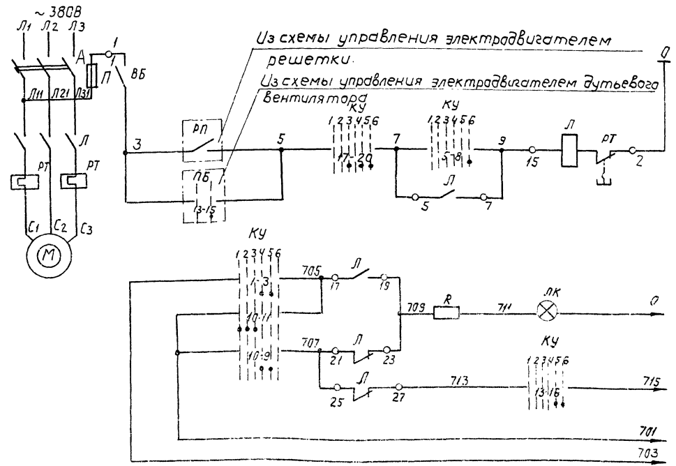
Схема подключения
