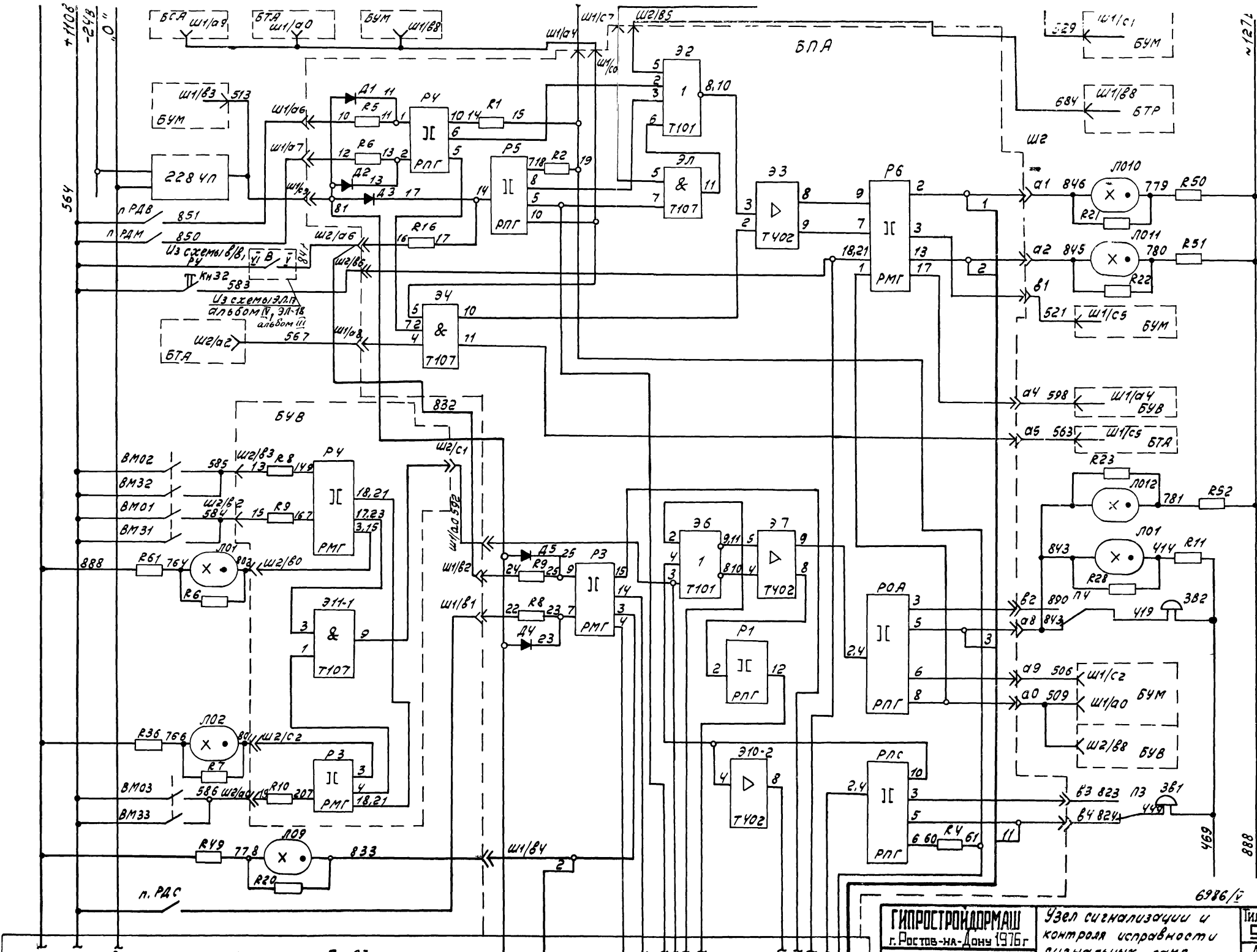
см. лист А-63 схема выполнена на листах А-61, А-62, А-63, А-64
