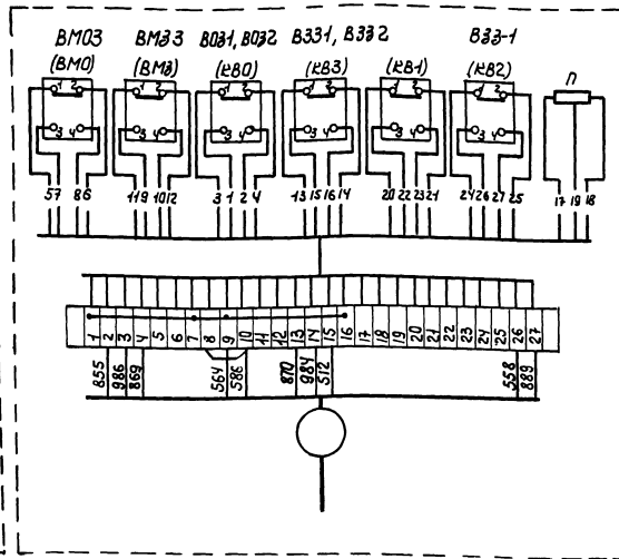
Задвижка магнетания ДЗН.
