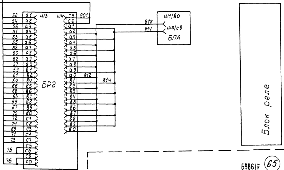
Схема выполнена на листах А-70, А-71, А-72
