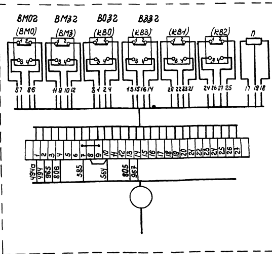
Диаграмма замыкания контактов конечных выключателей задвижек.
