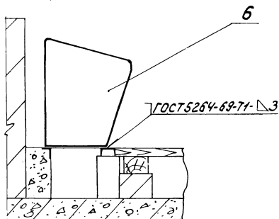
Б-Б повернуто M1:20
