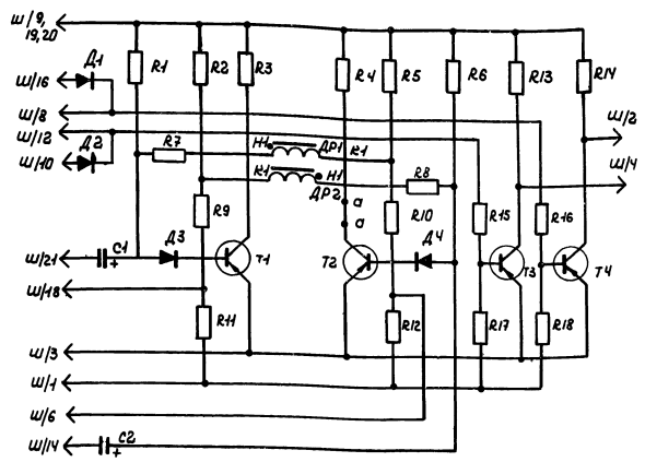
На данном листе представлена копия чертежа 6БХ401 62793 предприятия №А М-5878.
