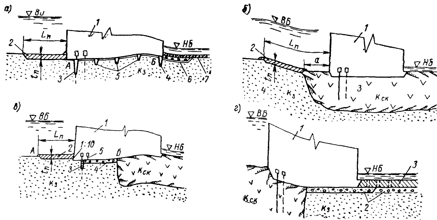
Рис. 6. Противофильтрационные устройства подземного контура для четырех типов тектонических трещин
