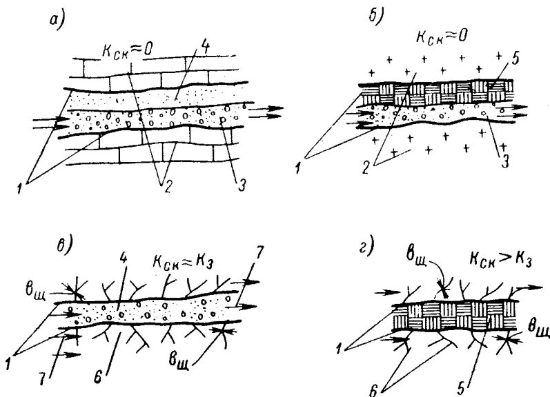
Рис. 2. Тектонические трещины (зоны дробления) с разным составом заполнителя
