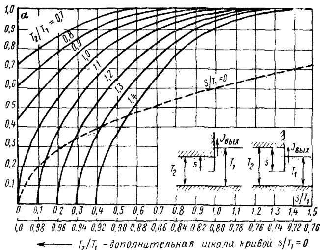
Рис. 14. График для определения коэффициента \alpha
