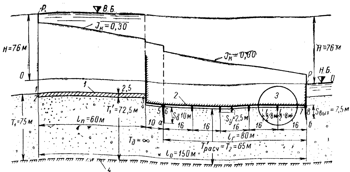
Рис. 12. Расчетная схема
