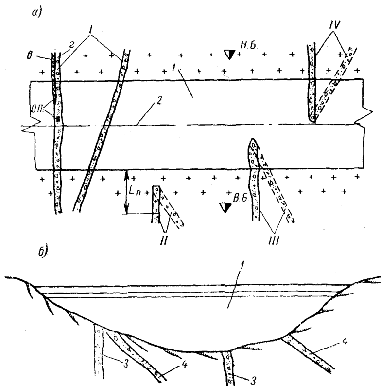
Рис. 1. Расположение тектонических трещин
