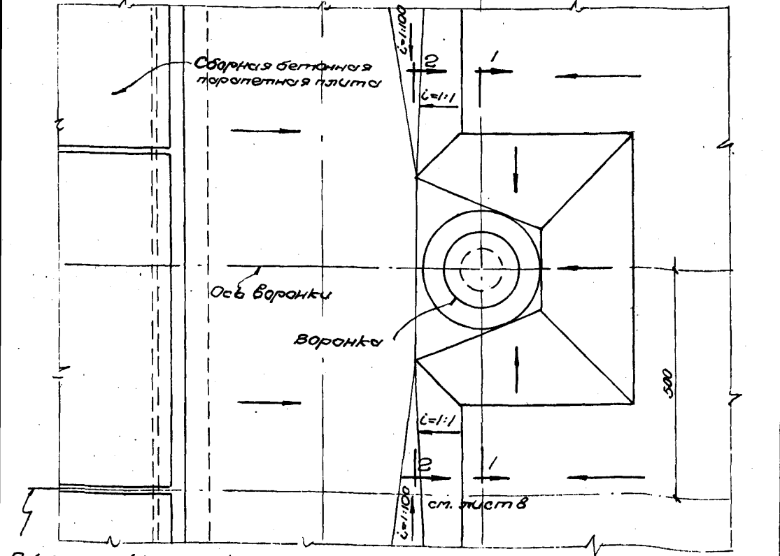
План ендовы
