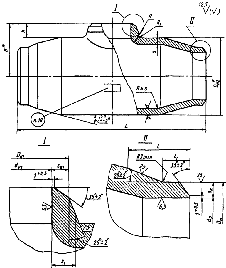
* Размеры для справок Черт. 4
