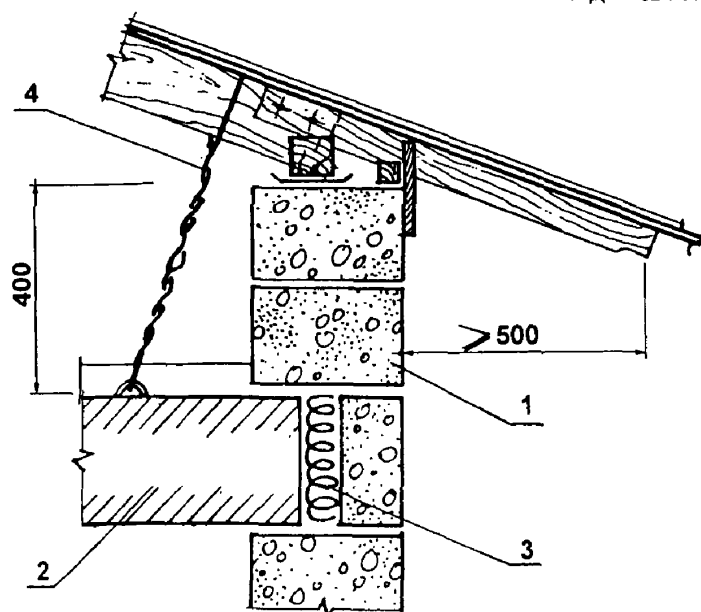
1 - Мелкий ячеистобетонный блок; 2 - Плита перекрытия; 3 - Утеплитель; 4 - Скрутка из стальной проволоки
