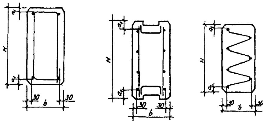
Рисунок 6.1 – Рекомендуемые варианты арматурных каркасов
