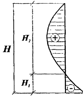
Рисунок 4.17 – Схема знакопеременной эпюры изгибающих моментов по высоте стены
