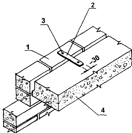
Рисунок 4.8 - Анкеровка наружной стены в ячеистобетонном перекрытии 1 - Мелкий ячеистобетонный блок, 2 - Полосовой металлический анкер; 3 – Стальной нагель; 4 - Ячеистобетонная плита перекрытия
