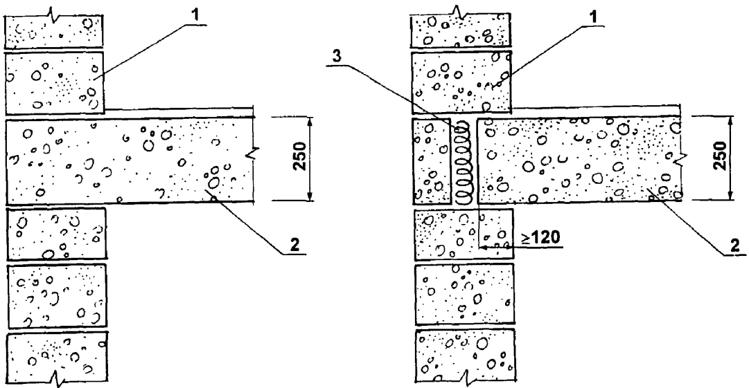
Рисунок 4.6 - Опираение деревянных балок перекрытия на наружную стену из мелких блоков
