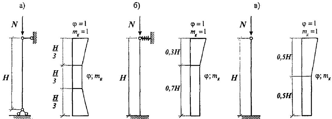
Рисунок 4.16 - Эпюры коэффициентов \varphi и m_g сжатых стен и столбов из ячеистобетонных мелких блоков а – шарнирно опертых на неподвижные опоры внизу и вверх; б – защемленных внизу и с упругой опорой вверх; в – защемленных внизу и свободных вверх.
