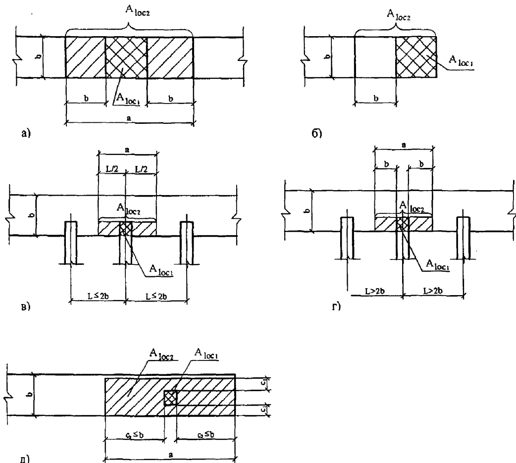
Рисунок 4.18 - Расчетные схемы для местного сжатия
