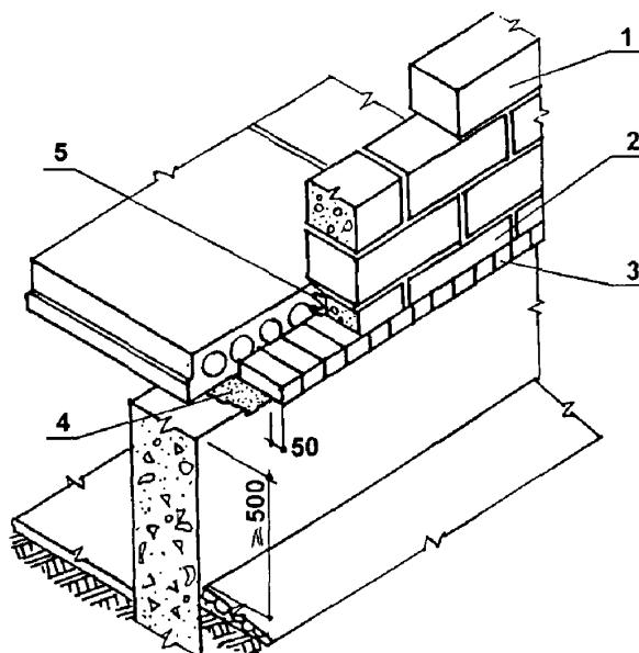
Рисунок 4.12 - Схема узла цоколя здания с опиранием первого ряда ячеистобетонных блоков на кирпичи
