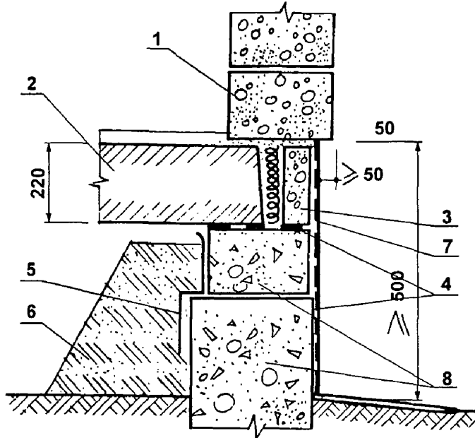
Рисунок 4.12 - Схема узла цоколя здания с опиранием первого ряда ячеистобетонных блоков на кирпичи
