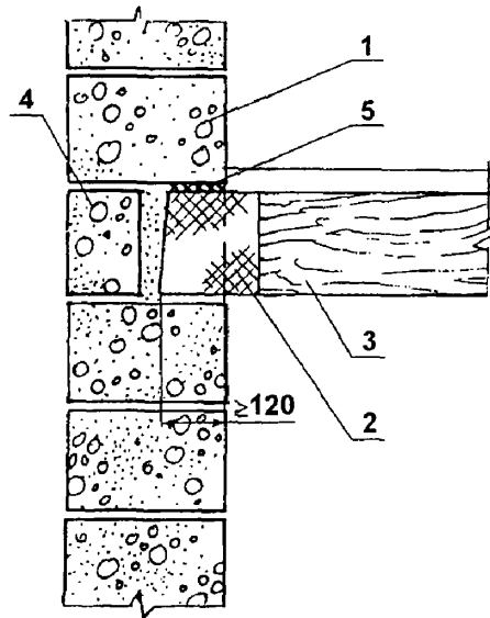
1 - Мелкий ячеистобетонный блок; 2 - Обертка толем; 3 - Балка деревянного перекрытия; 4 - Доборный блок; 5 - Асбестовая прокладка
