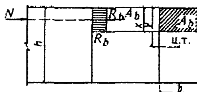
Рисунок 5.1 - Схема усилий и эпюра напряжений в сечении, нормальном к продольной оси внецентренно сжатого бетонного элемента, рассчитываемого по прочности без учета сопротивлений бетона растянутой зоны
