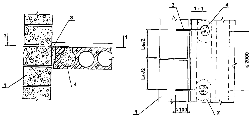
1 - Мелкий ячеистобетонный блок; 2 - Плита перекрытия; 3 - Стальная скоба диаметром 6 мм; 4 – Раствор Рисунок 4.9 - Анкеровка наружной стены к железобетонной плите перекрытия
