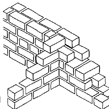
Рисунок 4.4в - Сопряжение наружной кладки толщиной в 2 однотипных блока и внутренней стены
