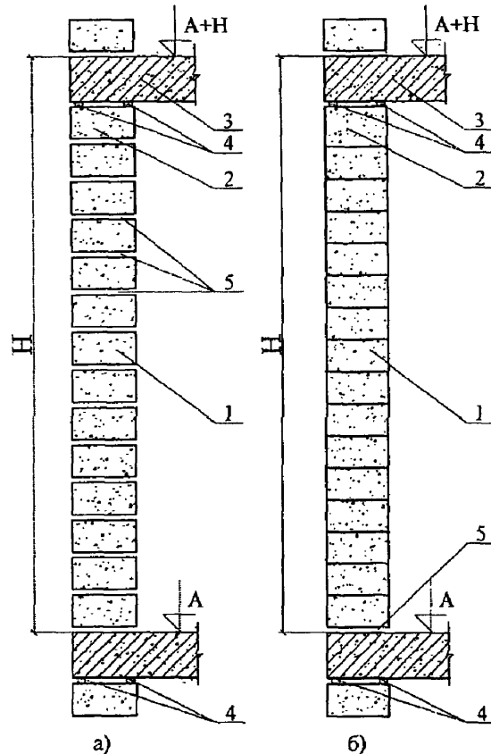
Рисунок 4.10 - Схема кладки наружных самонесущих с поэтажным опиранием стен из мелких ячеистобетонных блоков при ячеистобетонных перекрытиях а) блоки на растворе; б) блоки на клею
