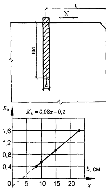
Рисунок 7.2 – График зависимости между несущей способностью забивного или вклеенного анкерного крепления и расстоянием «b» от грани панели
