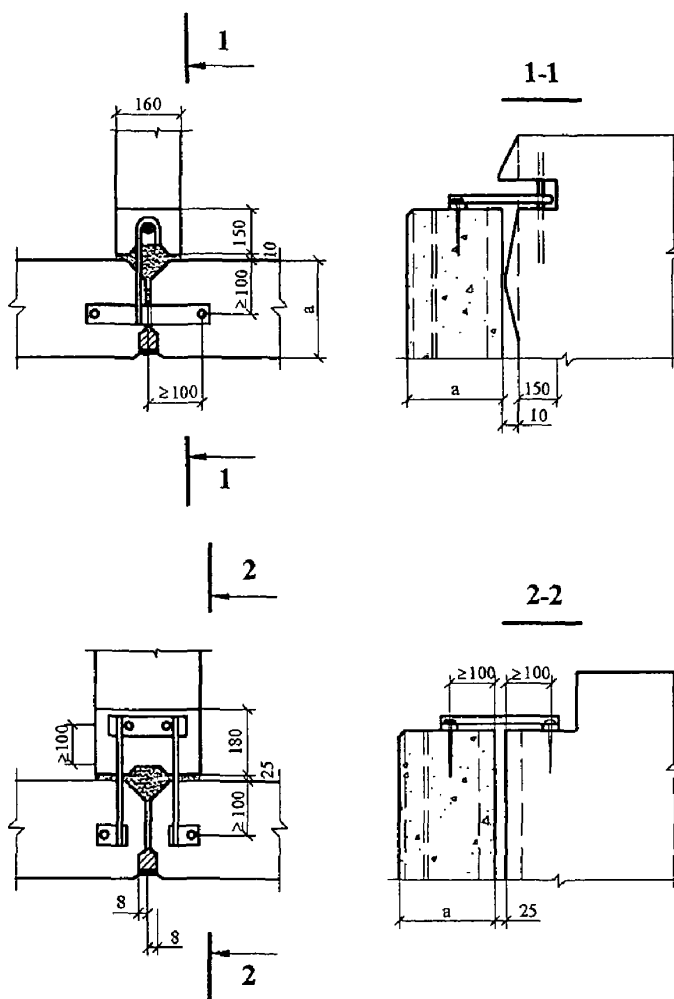
Рисунок 7.4 – Примеры узлов соединения и крепления
