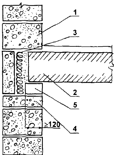
1 - Мелкий ячеистобетонный блок; 2 - Железобетонная плита перекрытия; 3 - Минераловатный утеплитель; 4 - Доборные блоки; 5 - Кирпич или бетон.
