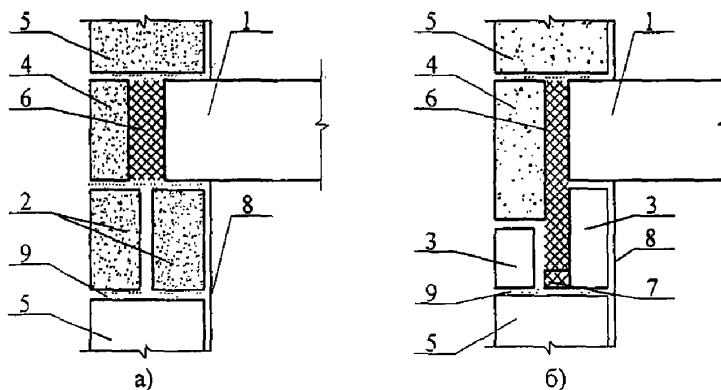
Рисунок 4.10 - Схема кладки наружных самонесущих с поэтажным опиранием стен из мелких ячеистобетонных блоков при ячеистобетонных перекрытиях а) блоки на растворе; б) блоки на клею
