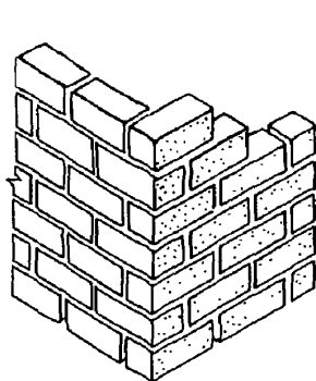
Рисунок 4.4а - Схема кладки угла здания
