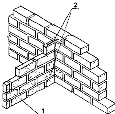
1 - Доборные блоки; 2 - Т – образный анкер 30*30*5, 84 Рисунок 4.4б - Примыкание перегородки к стене
