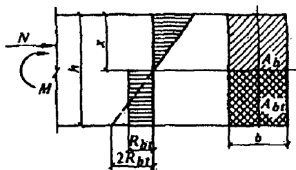
Рисунок 5.2 - Схема усилий и эпюра напряжений в сечении, нормальном к продольной оси изгибаемого (вицецепренно сжатого) бетонного элемента, рассчитываемого по прочности с учетом сопротивления растянутой зоны бетона
