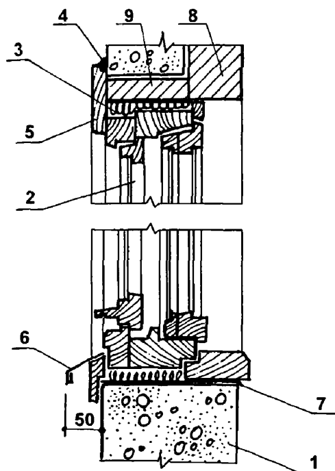
1 - Мелкий ячеистобетонный блок; 2 - Оконный блок; 3 - Просмоленная пакля; 4 - Герметизирующая мастика; 5 - Наличник; 6 - Слив; 7 - Толь; 8 - Несущая перемычка; 9 - Ненесущая перемычка (для опирания кладки, но не перекрытия).
