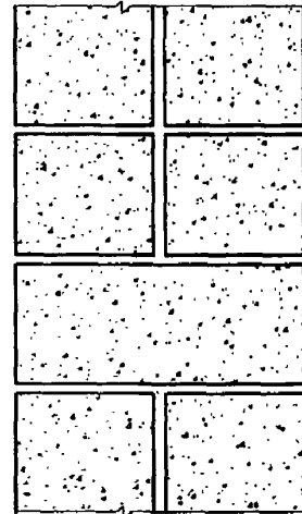
Рисунок 4.2б - Кладка наружных стен из однотипных ячеистобетонных блоков толщиной в 2 однотипных блока с перевязкой тычковыми блоками
