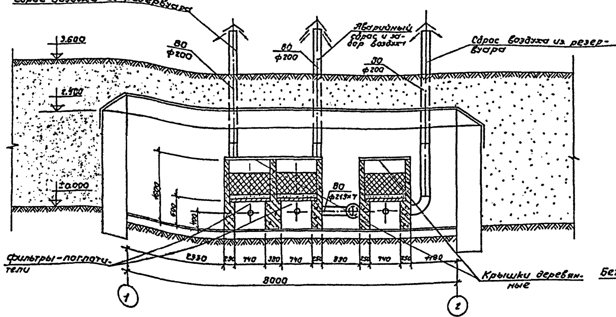
Разрез 1-1
