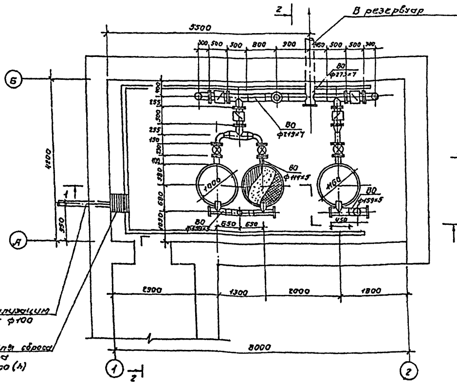
План на отн. 0.000
