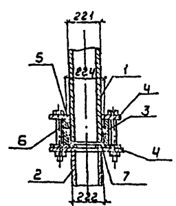
Узел А
