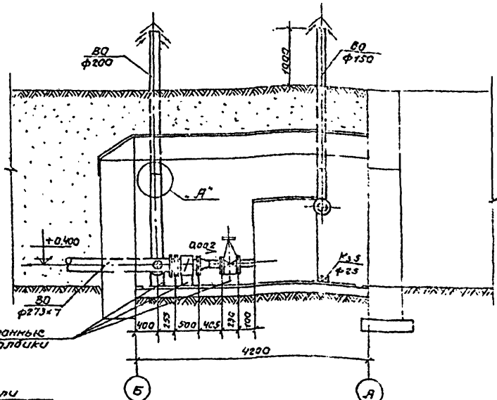
Разрез 2-2
