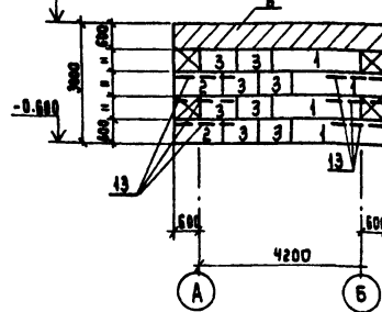
Раскладка блоков по оси 1
