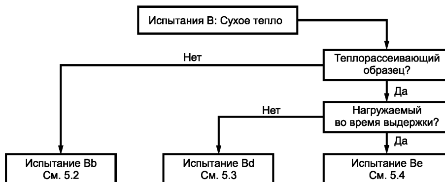
Рисунок 1 — Блок-схема испытаний В: Сухое тепло
