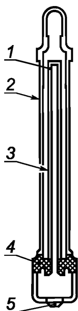
c – Вакуумный пробоотборник
