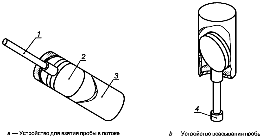
1 — кварцевая трубка; 2 — разъемная форма; 3 — картон; 4 — колпачок
