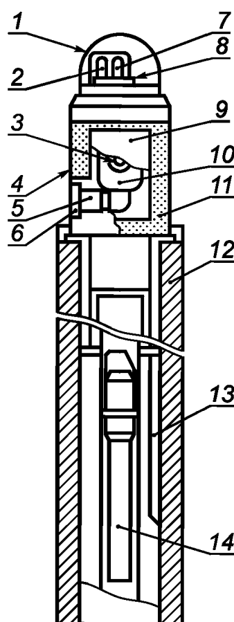
Рисунок А.4 — Пример погружаемого устройства для отбора проб жидкого чугуна из домны
