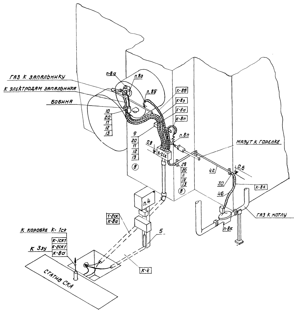
Электрические проводки по фронту котла
