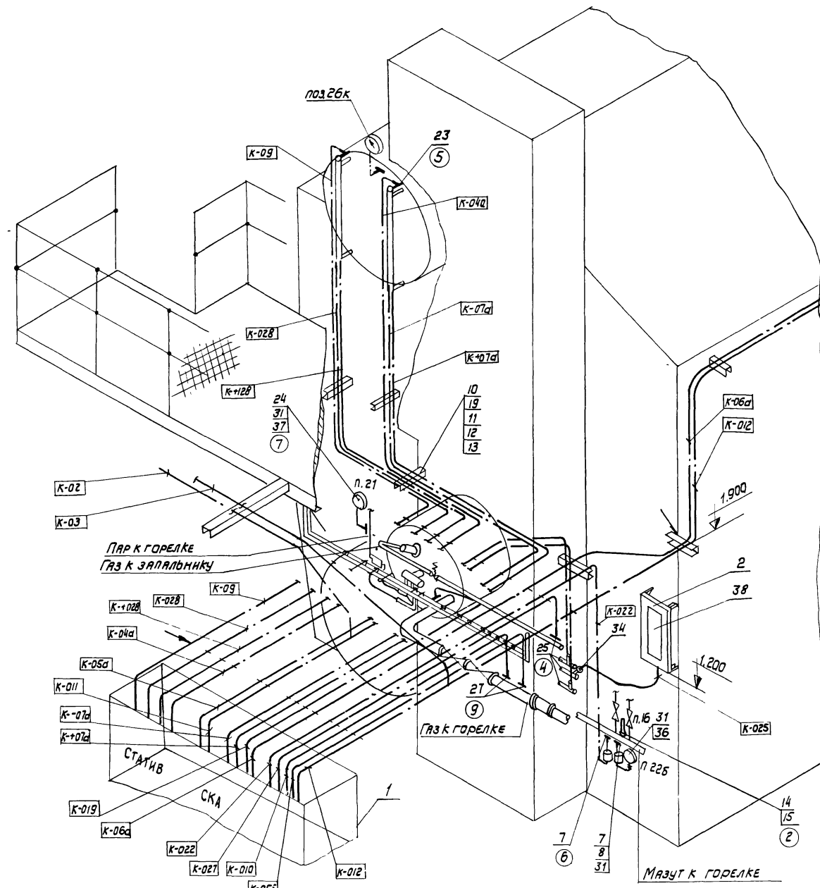
Трувные проводки по фронту котла
