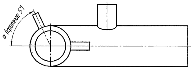
Рисунок 9 – Блок
