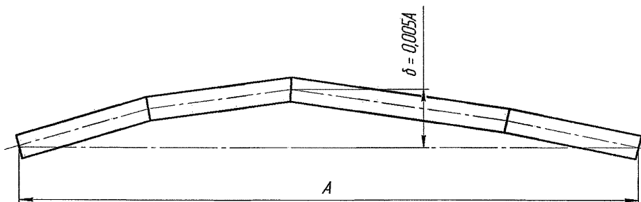
Рисунок 13 – Отклонение от номинального расположения оси блока
