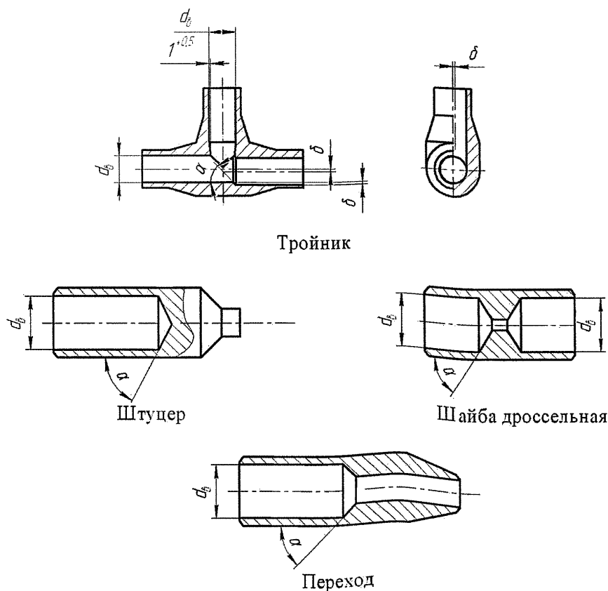
Рисунок 8 – Конусные расточки
