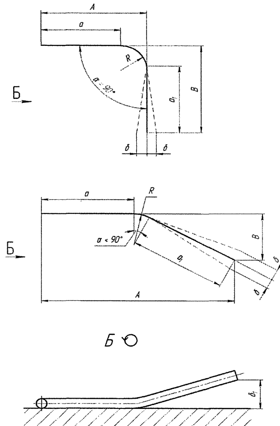
Рисунок 3 – Выход прямого участка из плоскостигиба
