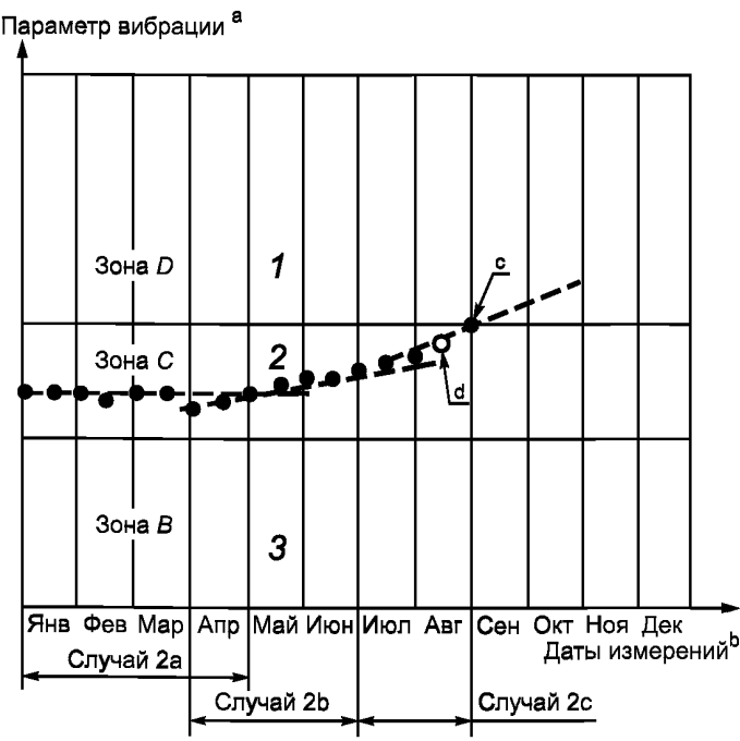
Рисунок 13 — Измерения широкополосной вибрации на вращающихся валах или корпусе машины. Вибрация вблизи уровня ПРЕДУПРЕЖДЕНИЕ
