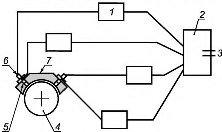
1 — устройства формирования данных; 2 — удаленное средство считывания результатов измерений; 3 — дополнительный выход для устройств записи и анализа данных; 4 — вал; 5 — датчики перемещения бесконтактного типа; 6 — датчики инерционного типа; 7 — корпус машины
