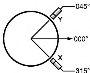
б) Нетрадиционное положение датчиков перемещений X и Y
