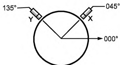
а) Положение датчиков перемещений X и Y
