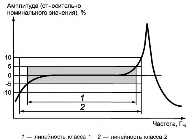
Рисунок 9 — Частотная характеристика измерительной цепи
