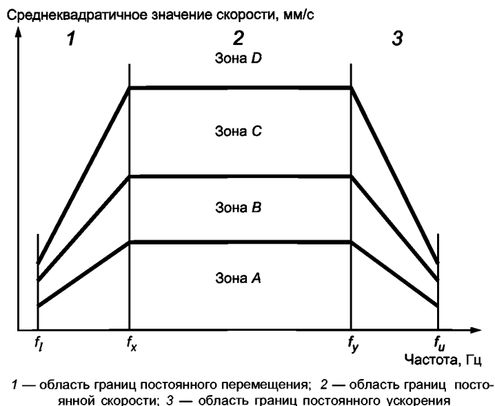
Рисунок 11 — Зоны вибрационного состояния
